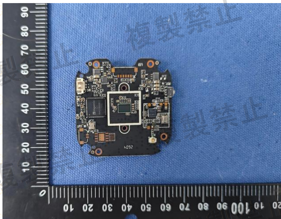
EUT Photo
