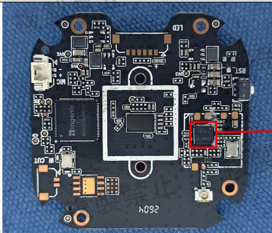
EUT Photo
