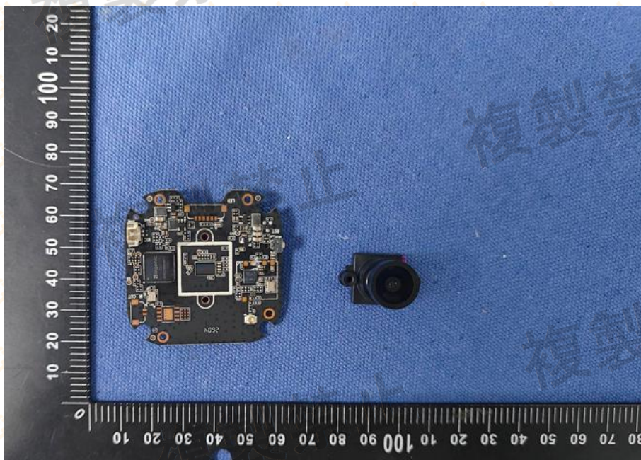
EUT Photo
