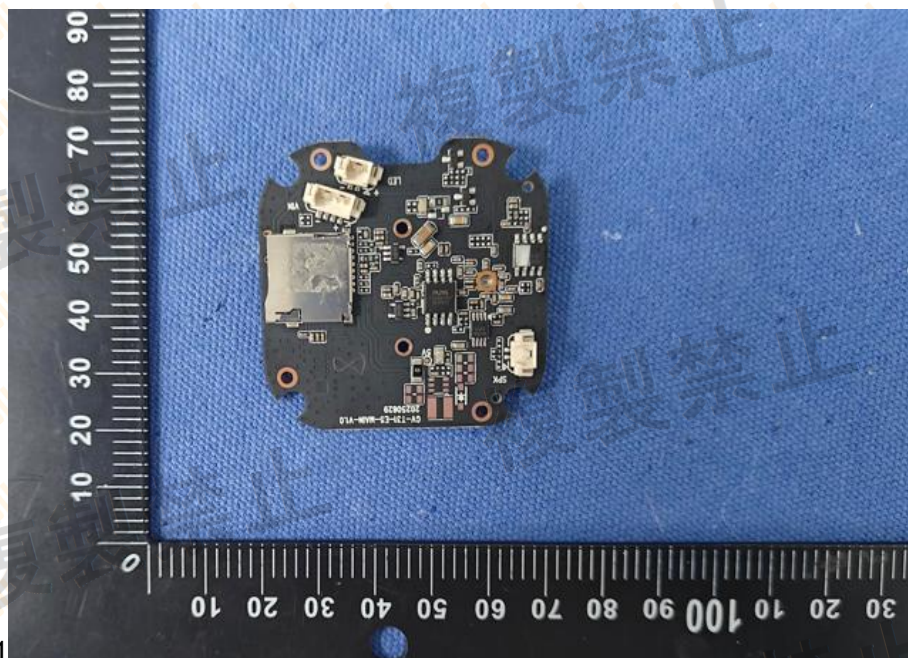
EUT Photo
