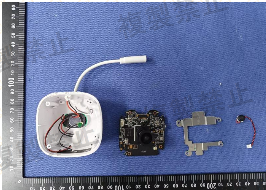
EUT Photo
