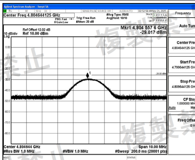
NTNV_DH5_Ant1_2402_4804.64
