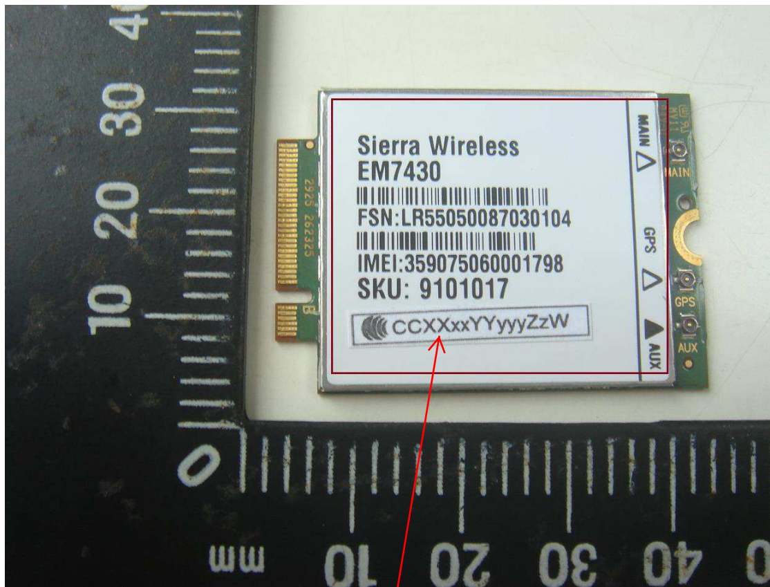
AirPrime EM7430(紅框為 NCC ID 位置)正面照
