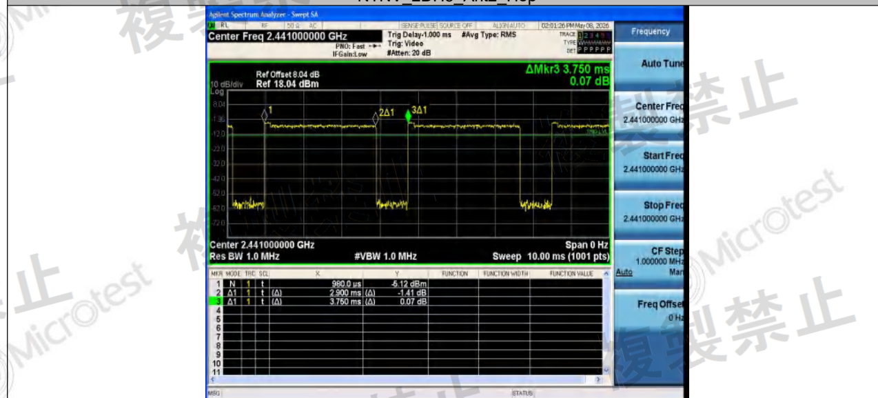
NTNV_2DH5_Ant2_Hop
