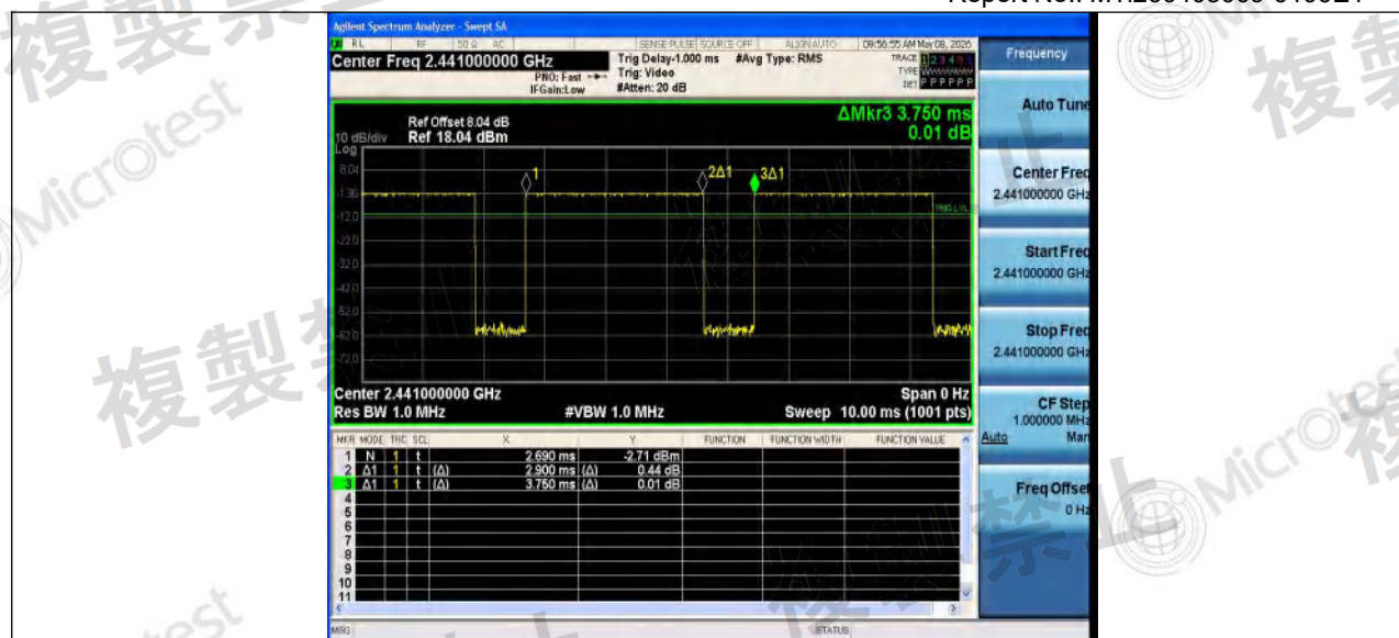
NTNV_DH5_Ant2_Hop
