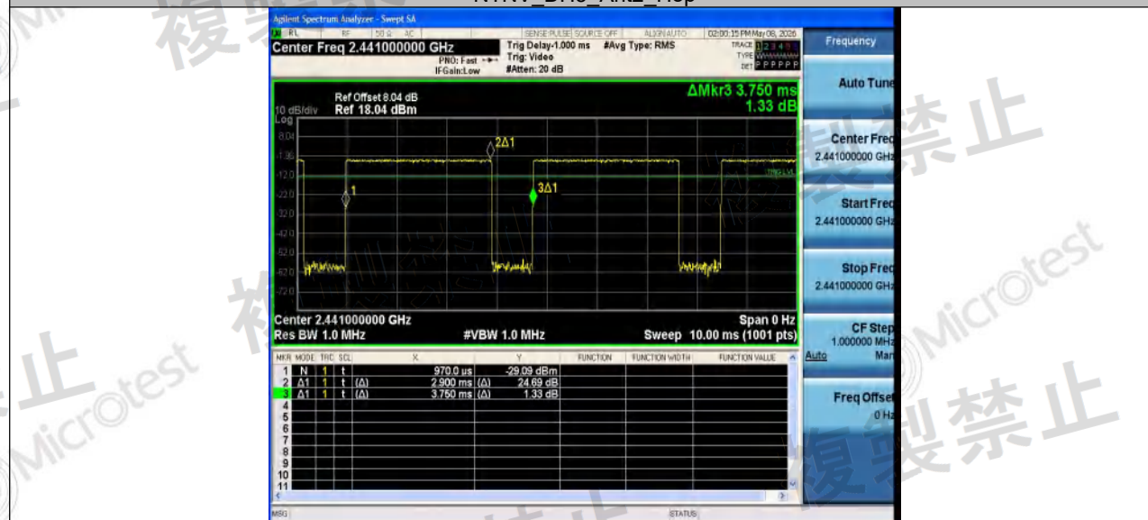
NTNV_DH5_Ant2_Hop
