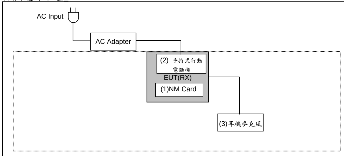
幅射干擾測試配置_EUT RX
