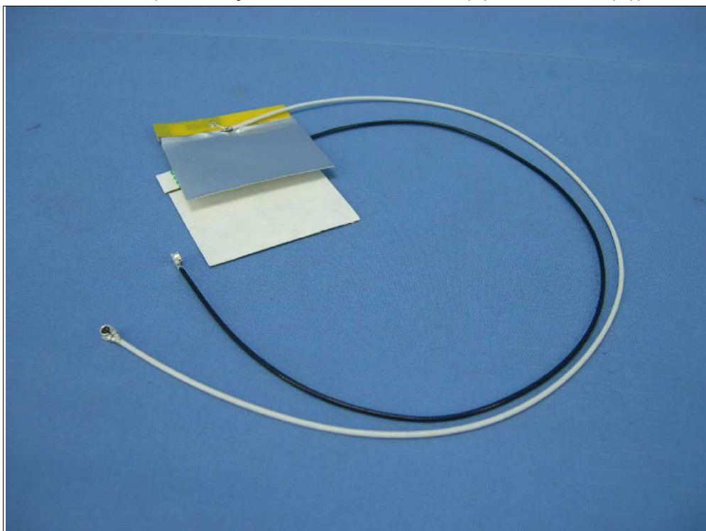
天線 81 (Brand: Tyco / Model: 2023644-1 (L), 2023645-1 (R))
