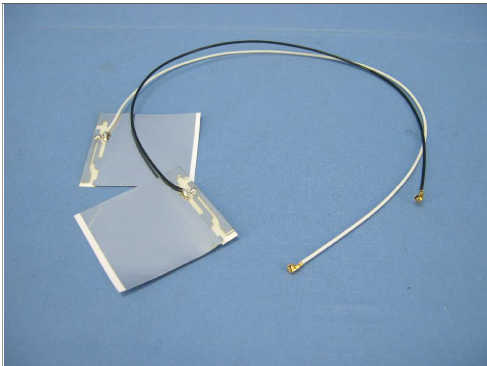
天線 80 (Brand: Yageo / Model: CAN4313 812 012501B (Main), CAN4313 812 022501B (Aux))
