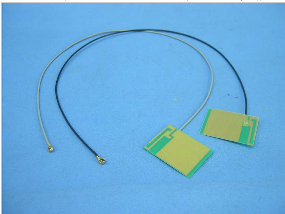
天線 103 (Brand: Hitachi / Model: HFT65 (Tx1), HFT65 (Tx2))
