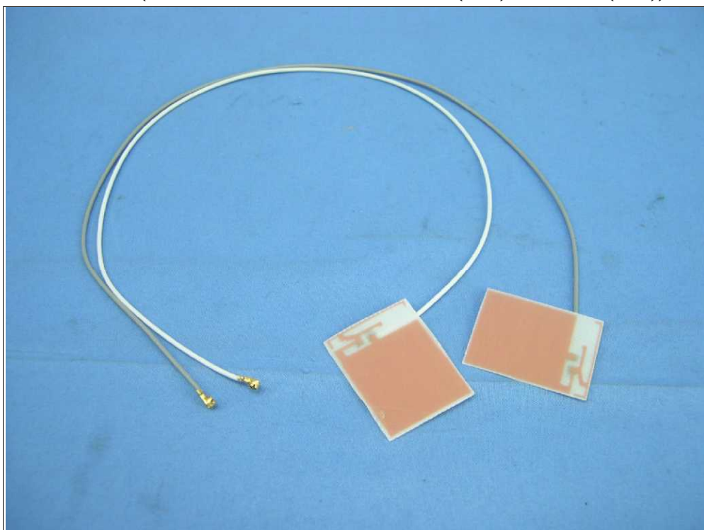
天線 100 (Brand: Hitachi / Model: HBY052 (Tx1), HBY052 (Tx2))
