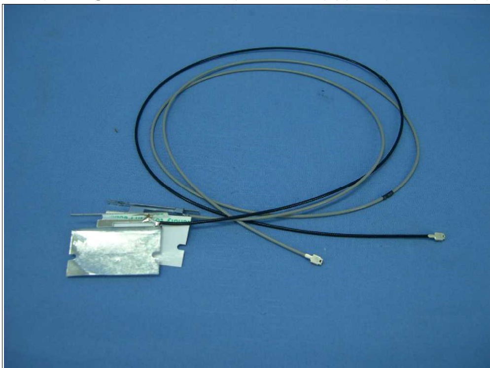
天線 83 (Brand: SpeedTech / Model: J10 (22G643000-10) (L), J10 (22G643000-10) (R))
