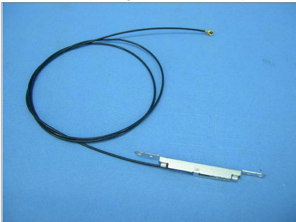
天線 88 (Brand: wgt / Model: TW18LWIP101+A)
