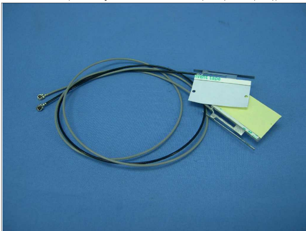
天線 70 (Brand: SpeedTech / Model: G10 (Main), G10 (Aux))
