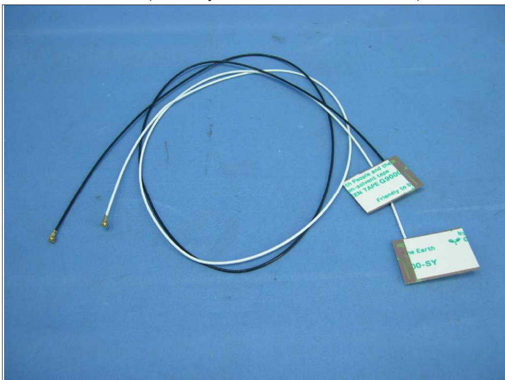
天線 92 (Brand: Tyco / Model: TBN005, TBN006)
