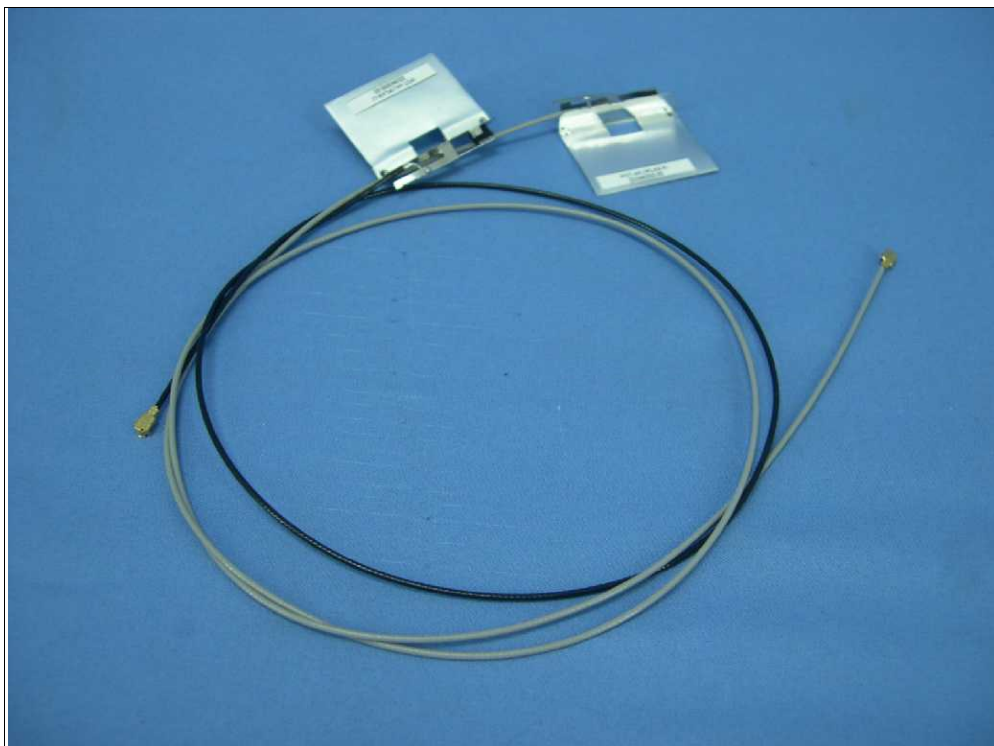
天線 72 (Brand: wgt / Model: A41/A40-L 22G645000-00, A41/A40-R 22G660020-00)
