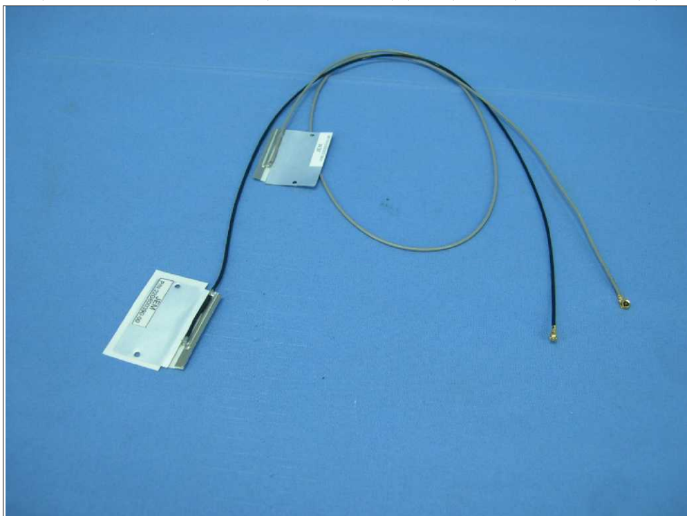
天線 73 (Brand: JEM / Model: U42 (22G600390-00) (Main), U42 (22G600540-30) ( Aux))
