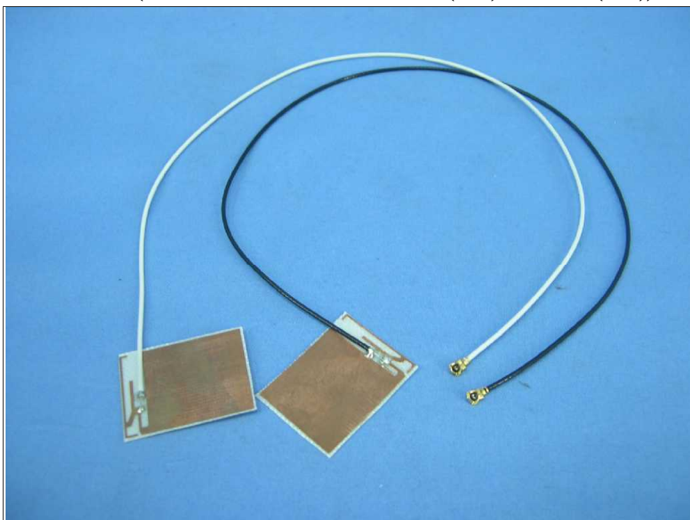
天線 101 (Brand: Hitachi / Model: HBY061 (Tx1), HBY061 (Tx2))
