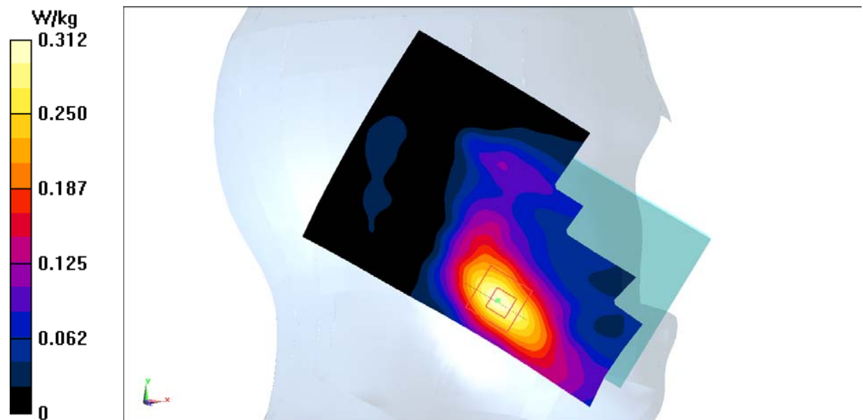
Fig.11 WCDMA1900
