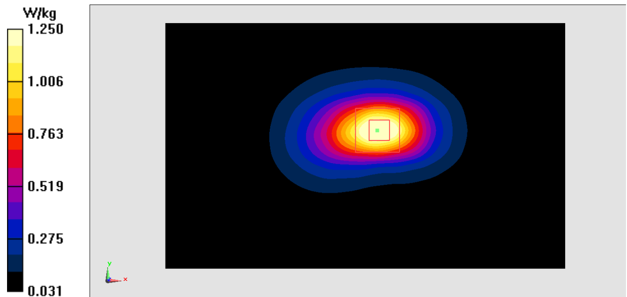
Fig.12 WCDMA1900
