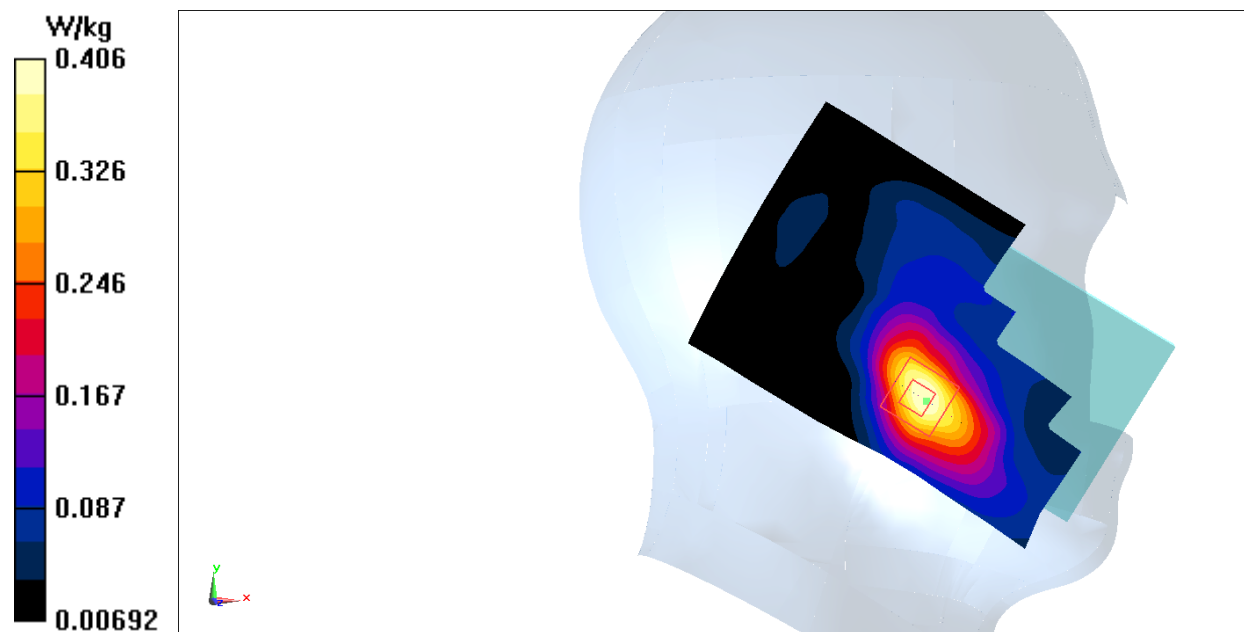
Fig.8 1700MHz
