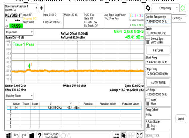
TX 2496.5MHz~12.5GHz BLE 500k 2402MHz
