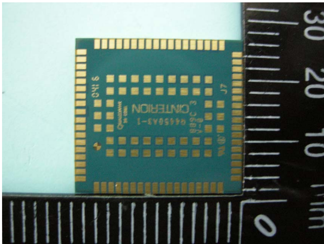
相片三：主機板背面照
