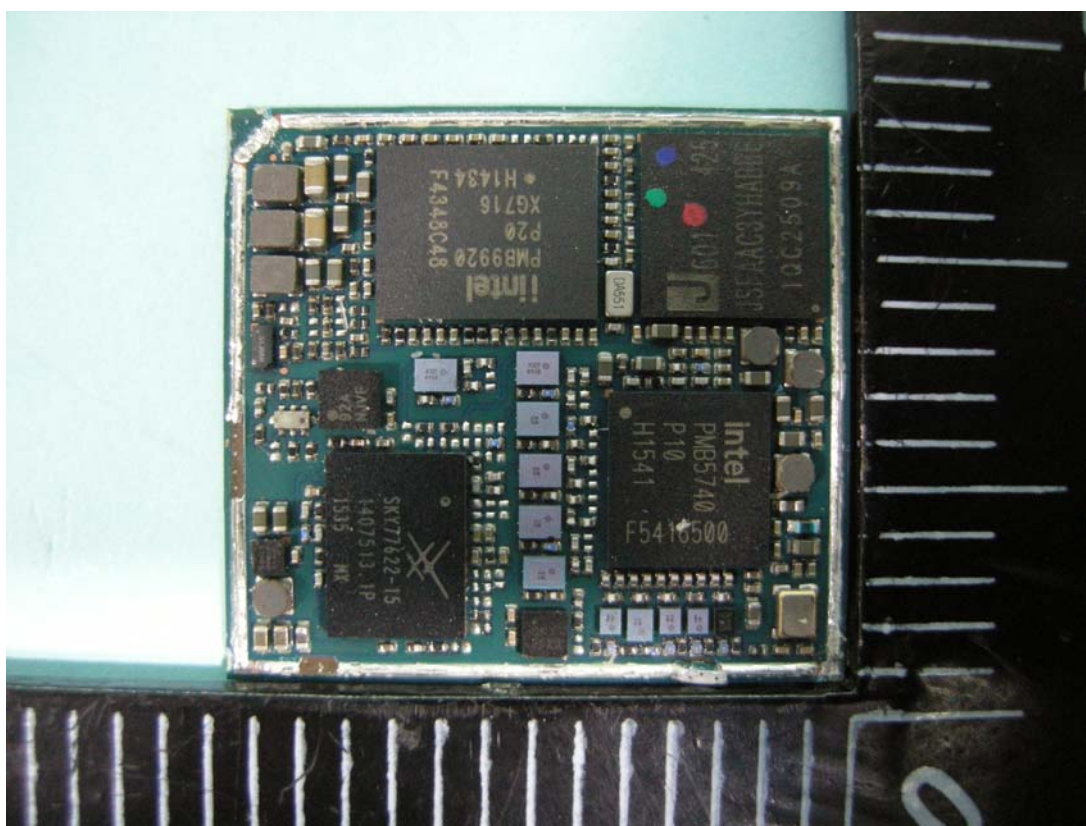
相片二：主機板內部照
