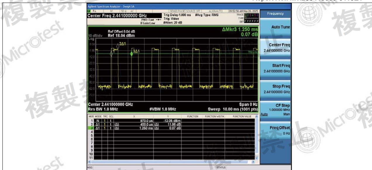
NTNV_2DH3_Ant1_Hop
