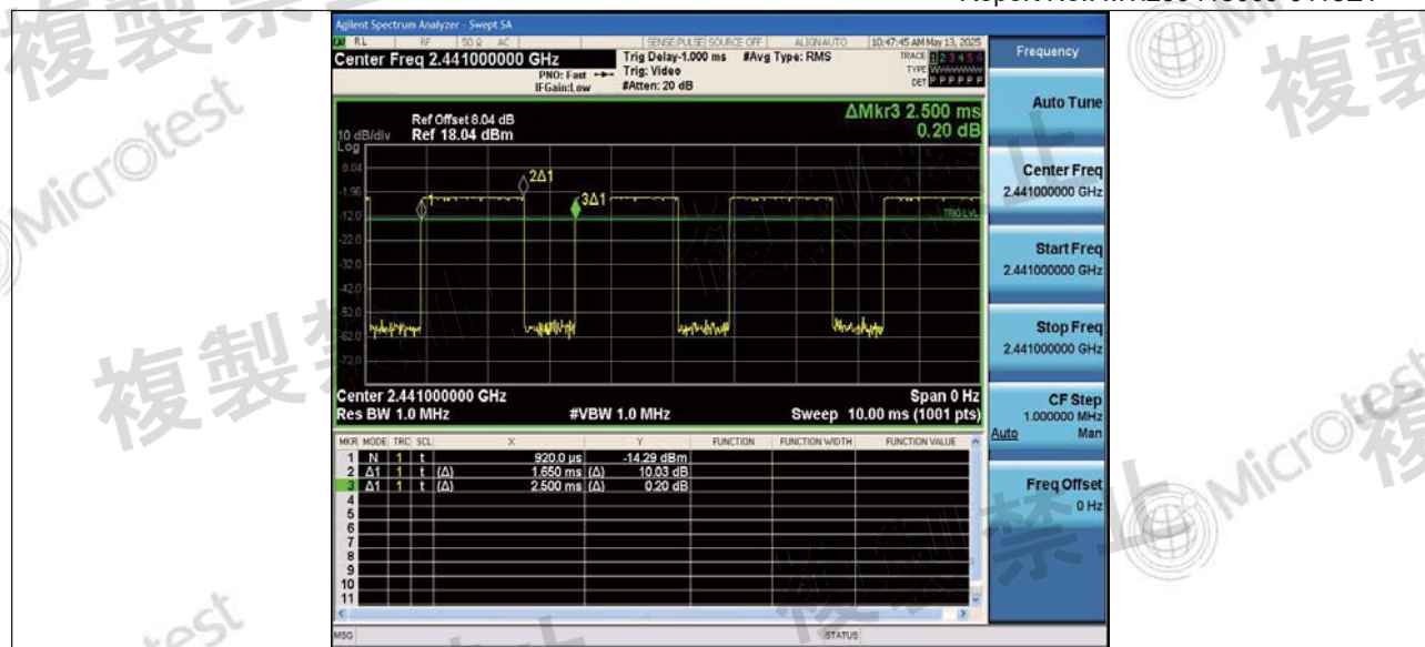
NTNV_DH3_Ant2_Hop
