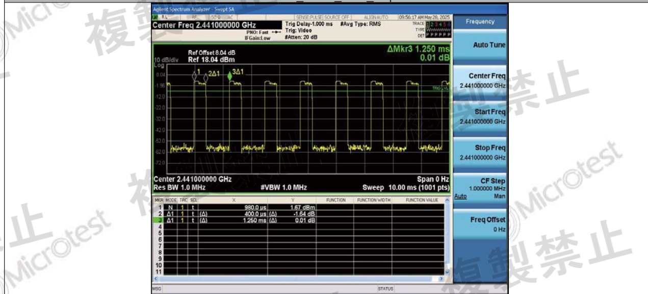
NTNV_3DH3_Ant1_Hop
