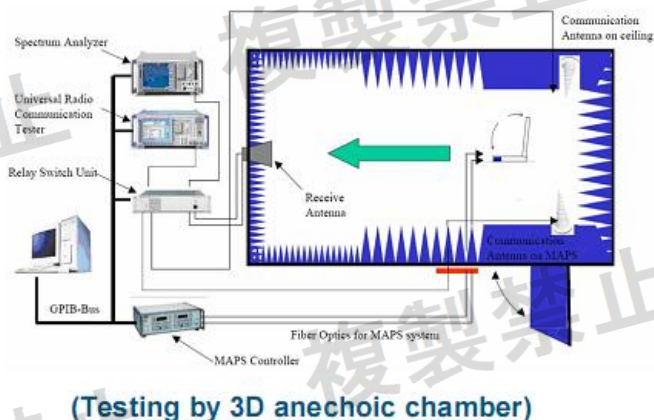
图 1 Test topology
