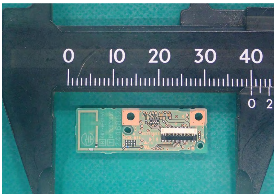
EUT Photo 5 )
