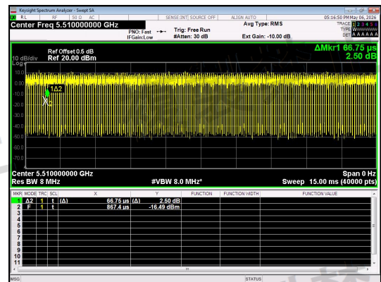
NT/NV_Antenna 1_IEEE 802.11ax_40_Channel 102_RU&Index SU
