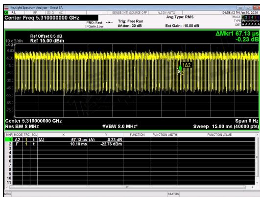
NT/NV_Antenna 0_IEEE 802.11ax_40_Channel 62_RU&Index SU
