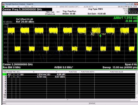
NT/NV_Antenna 0_IIEEE 802.11ax_20_Channel 52_RU&Index SU
