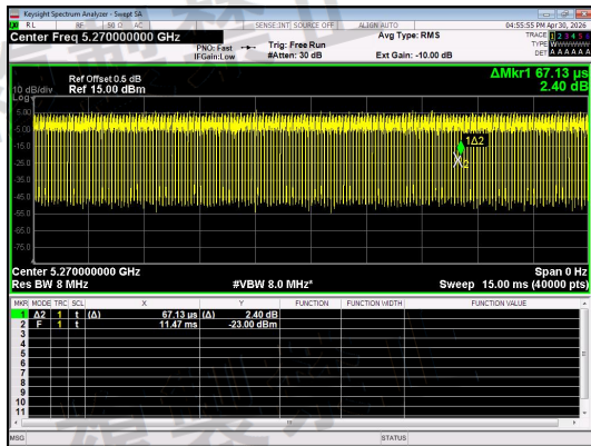
NT/NV_Antenna 0_IEEE 802.11ax_40_Channel 54_RU&Index SU
