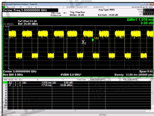
NT/NV_Antenna 0_ IEEE 802.11ax_20_Channel 120_RU&Index SU
