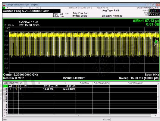
NT/NV_Antenna 0_IIEEE 802.11ax_40_Channel 46_RU&Index SU
