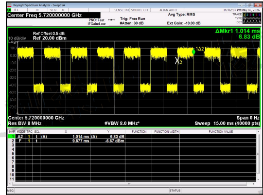
NT/NV_Antenna 1_IIEEE 802.11ax_20_Channel 144_RU&Index SU
