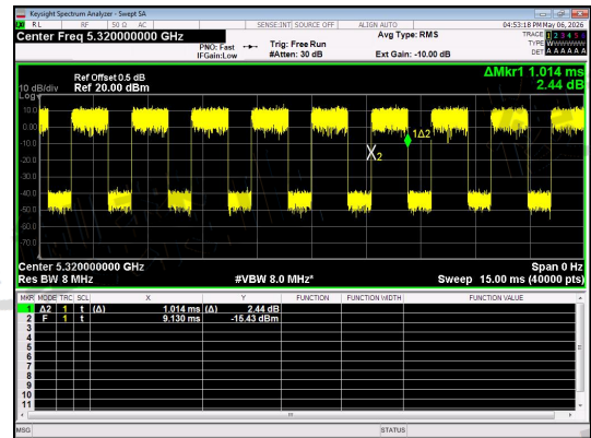
NT/NV_Antenna 1_ IEEE 802.11ax_20_Channel 64_RU&Index SU
