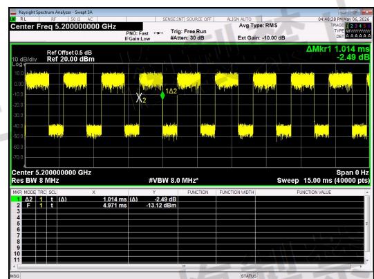
NT/NV_Antenna 1_IIEEE 802.11ax_20_Channel 40_RU&Index SU
