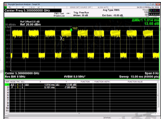
NT/NV_Antenna 1_IIEEE 802.11ax_20_Channel 60_RU&Index SU
