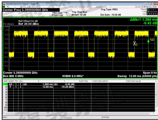
NT/NV_Antenna 0_ IEEE 802.11n_20_Channel 52
