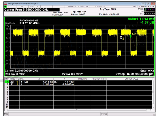
NT/NV_Antenna 1_IIEEE 802.11ax_20_Channel 48_RU&Index SU
