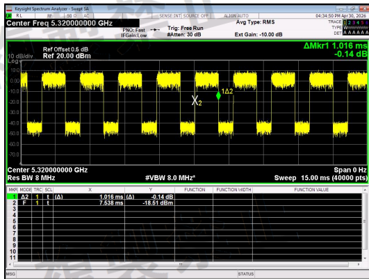
NT/NV_Antenna 0_ IEEE 802.11ax_20_Channel 64_RU&Index SU
