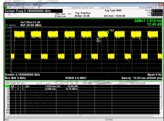
NT/NV_Antenna 1_IIEEE 802.11ax_20_Channel 36_RU&Index SU
