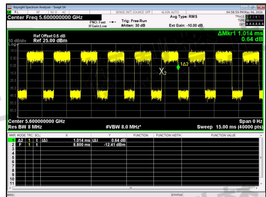
NT/NV_Antenna 1_ IEEE 802.11ax_20_Channel 120_RU&Index SU
