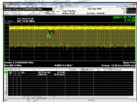
NT/NV_Antenna 1_IEEE 802.11ax_40_Channel 62_RU&Index SU
