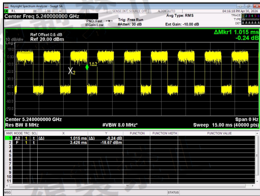
NT/NV_Antenna 0_IIEEE 802.11ax_20_Channel 48_RU&Index SU
