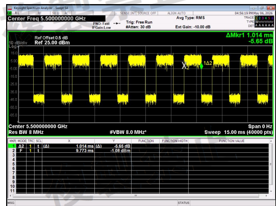
NT/NV_Antenna 1_ IEEE 802.11ax_20_Channel 100_RU&Index SU
