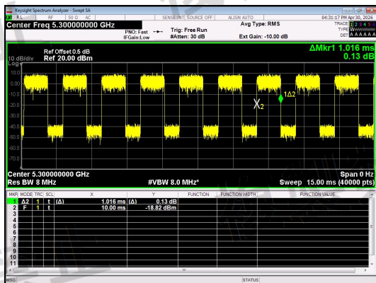
NT/NV_Antenna 0_IIEEE 802.11ax_20_Channel 60_RU&Index SU
