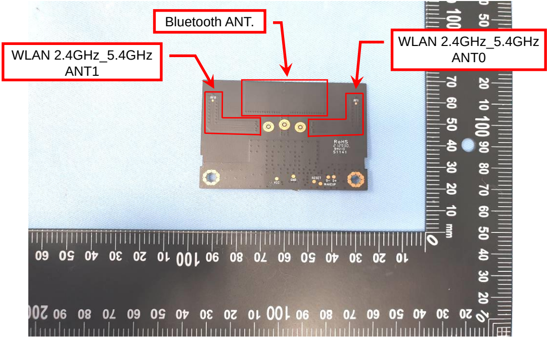
EUT Photo (2)
