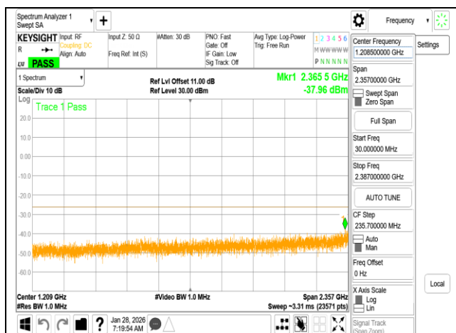
802.11b 20MHz Chain0 2412MHz Range1
