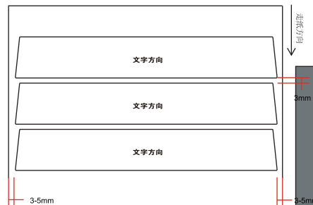
走纸示意图：
