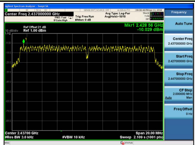
802.11 n-20M CH06 (2437MHz) (SISO)
