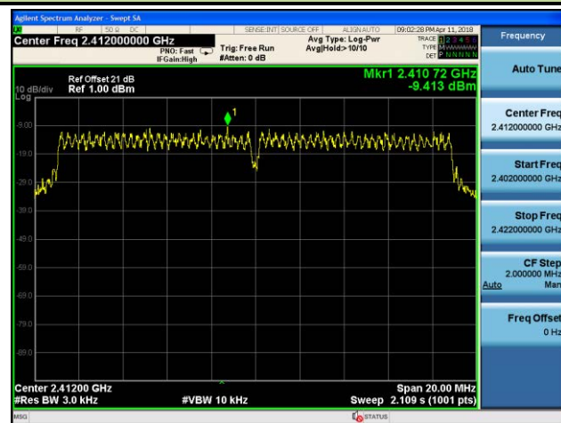
802.11 n-20M CH01 (2412MHz) (SISO)
