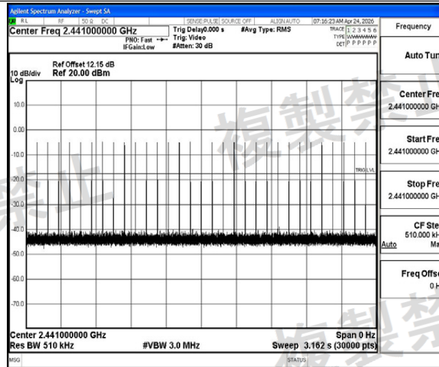
NTHV-2DH1-Ant1-Hop-PASS
