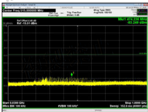
802.11ac20 CH: 5200MHz, 30MHz~1GHz
