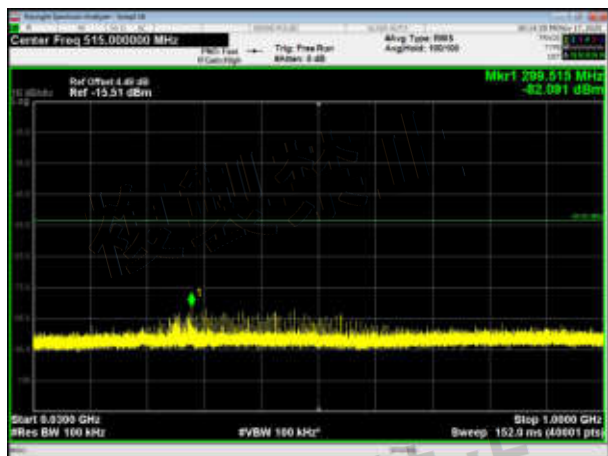
802.11a CH: 5200MHz, 30MHz~1GHz
