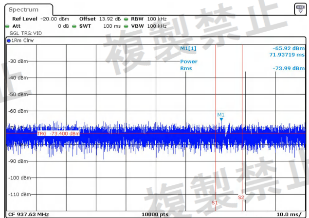
NTNV-11AC20-Ant2-5200-30~1000-PASS
