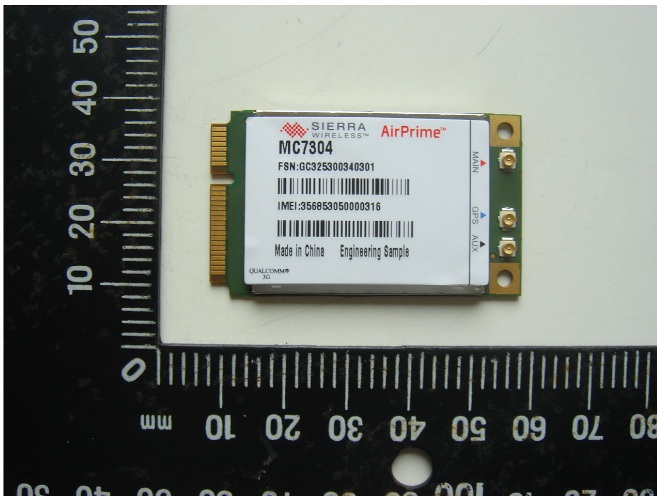
AirPrime MC7304 正面照
