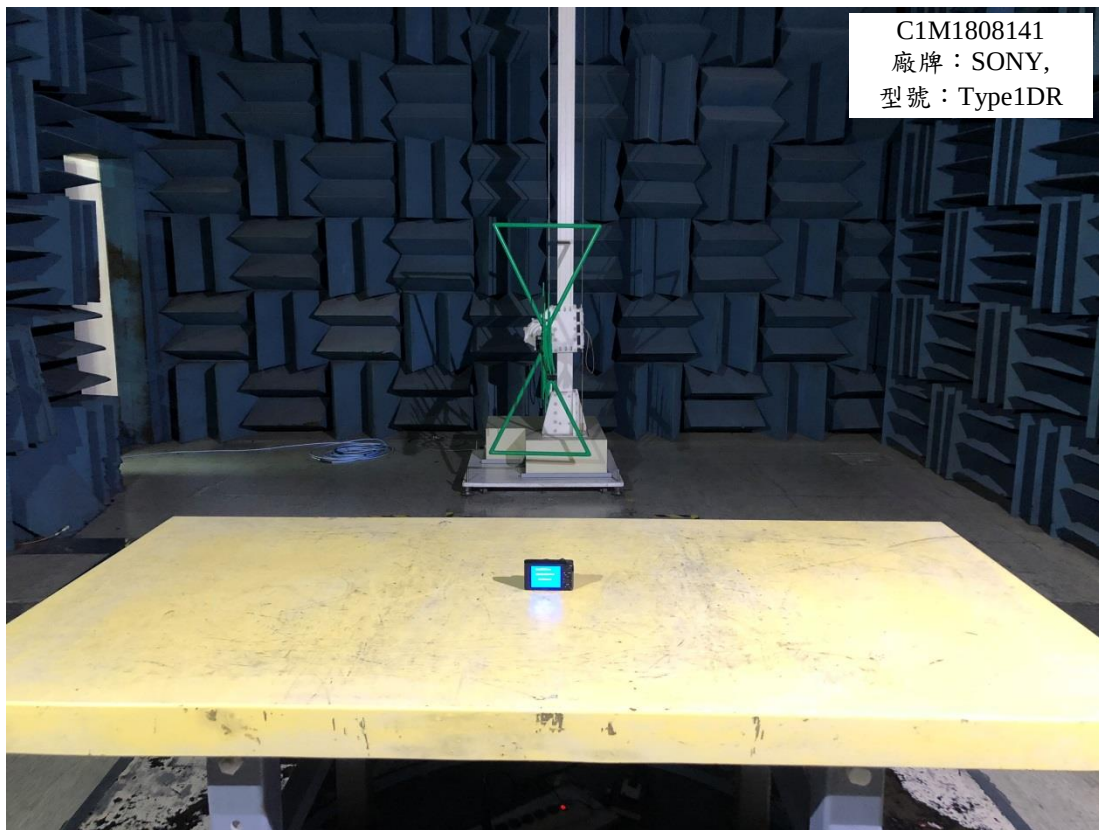
單機-站立
