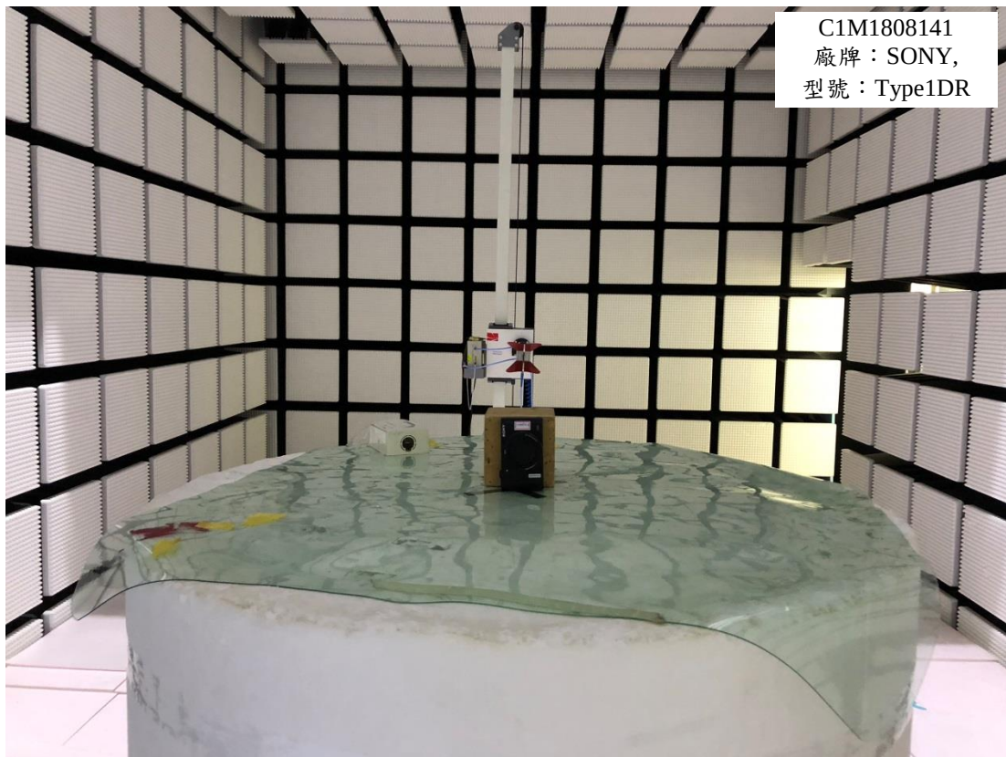
單機-側立
