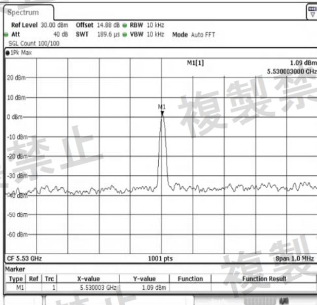
NTNV-11AC80SISO-Ant1-5530-PASS
