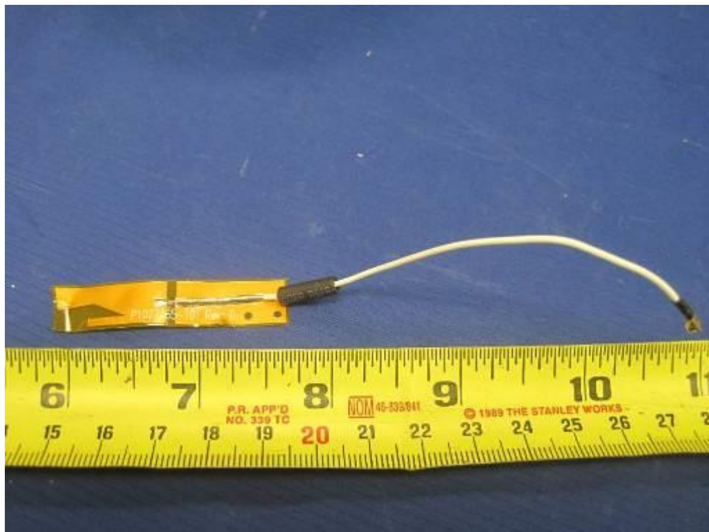
EUT – Antenna
