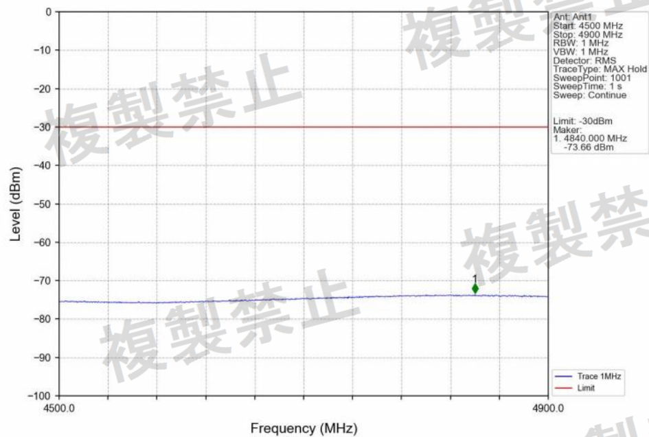
Band3 5MHz QPSK_LCH_1712.5MHz_RB_1_24_NTNV 25/25 4500-4900MHz Limit:-30
