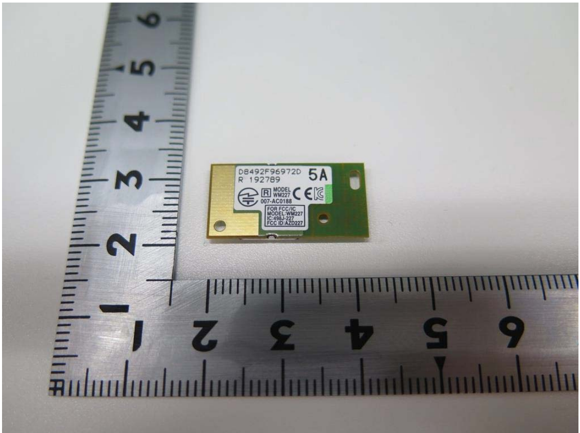
WiFi Module
