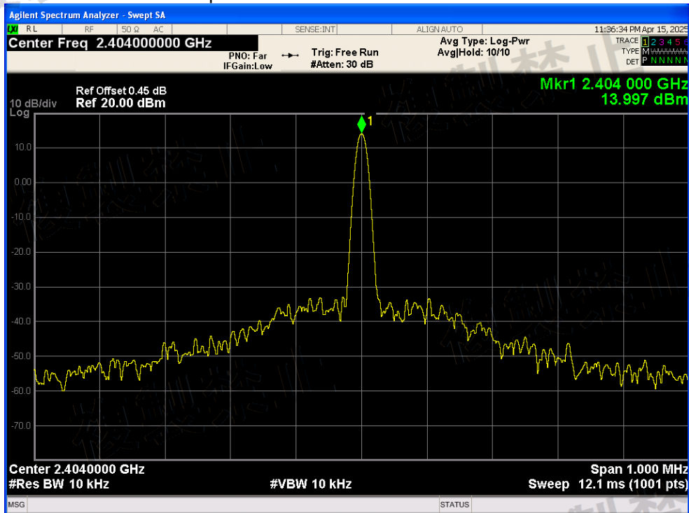
Freq. Error NVNT BLE 2M 2404MHz Ant1
