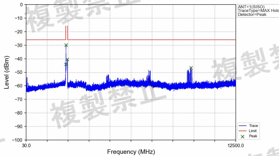
8DPSK 3DH5 HOPP_Ant1_NTNV
