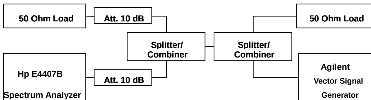
校驗架構圖
