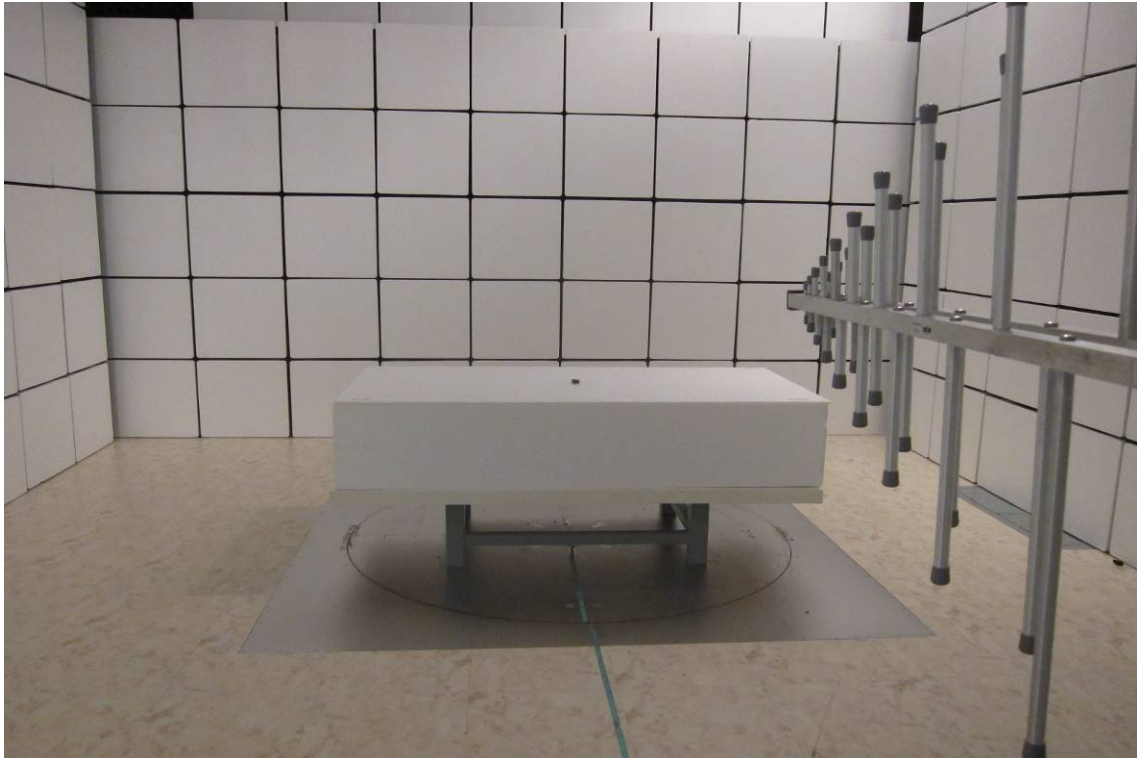
輻射干擾測試照片
