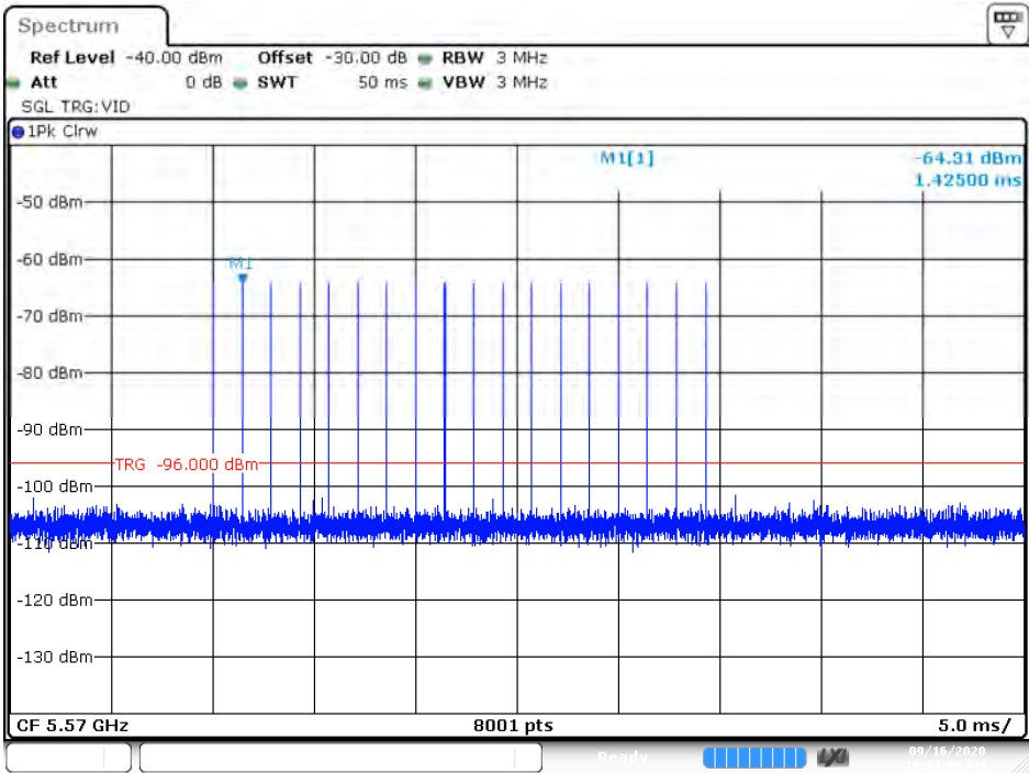
雷達測試信號 Type 0 校驗圖 for 5570MHz
