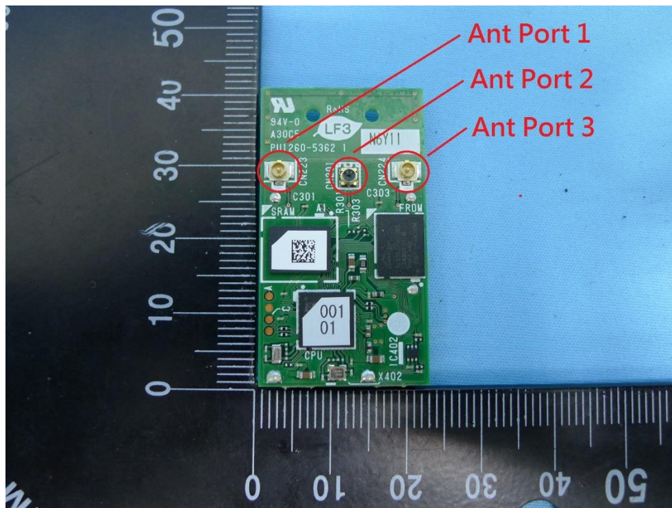
(1) 待測物照片
