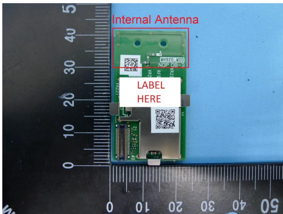
(2) 待測物照片
