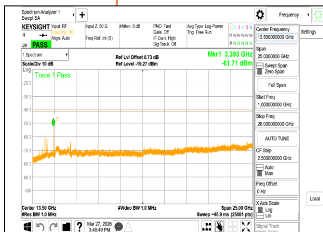
VLP 802.11be 80MHz Chain1 5985MHz Range2
