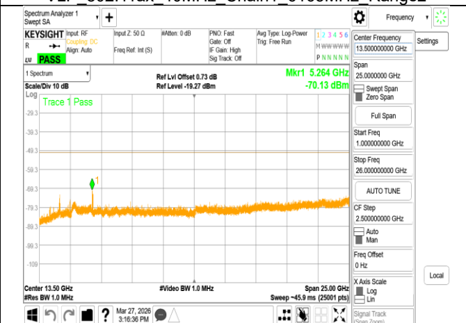
VLP 802.11ax 40MHz Chain1 6405MHz Range2
