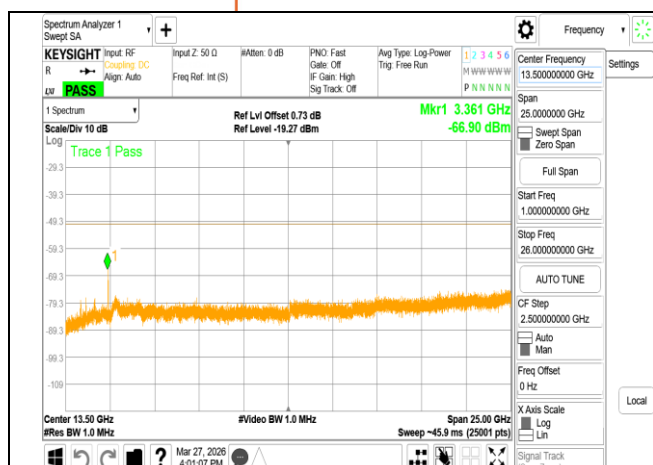
VLP_802.11be_160MHz_Chain0_6185MHz_Range2
