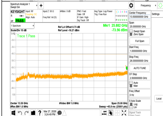
VLP 802.11ax 80MHz Chain1 6385MHz Range2
