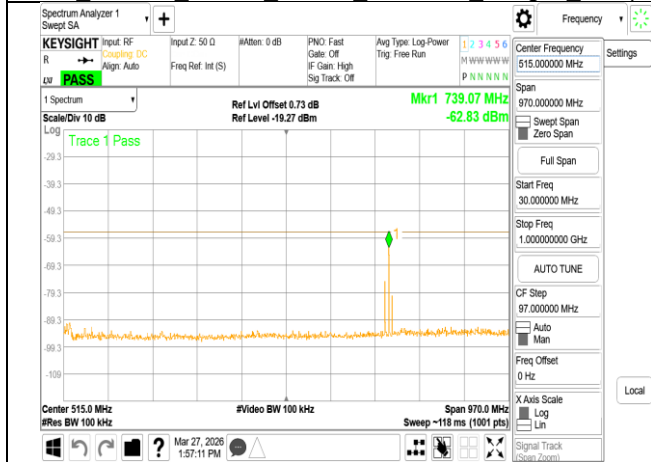
VLP 802.11n 40MHz Chain1 5965MHz Range1
