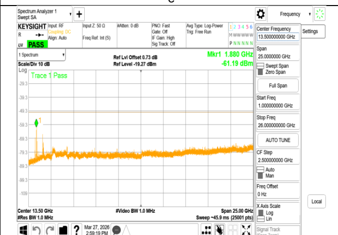
VLP_802.11ac_160MHz_Chain1_6345MHz_Range2
