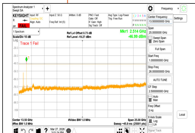
VLP 802.11ax 20MHz Chain0 5955MHz Range2
