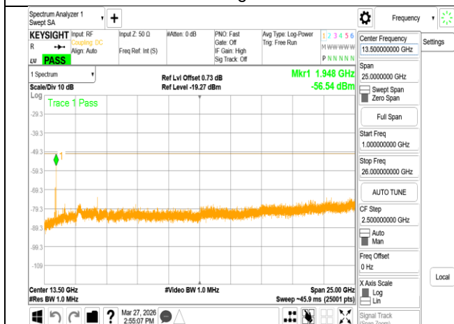
VLP_802.11ac_160MHz_Chain0_6185MHz_Range2
