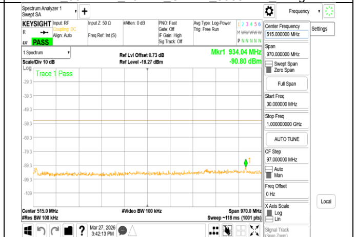
VLP 802.11be 40MHz Chain1 6165MHz Range1
