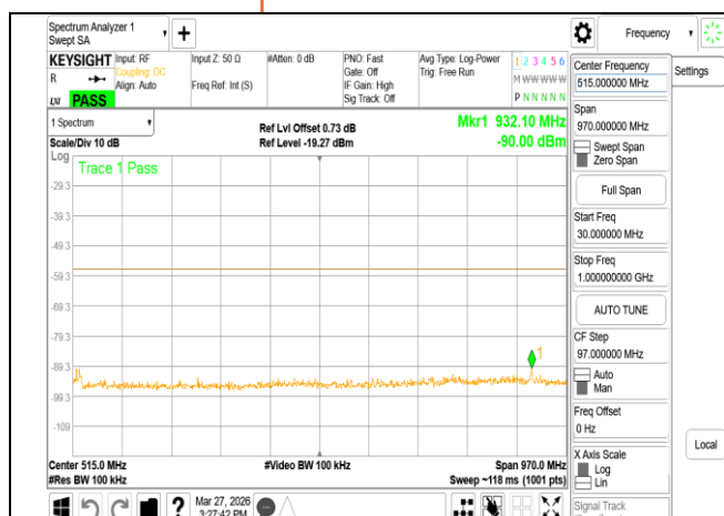
VLP_802.11ax_160MHz_Chain1_6185MHz_Range1
