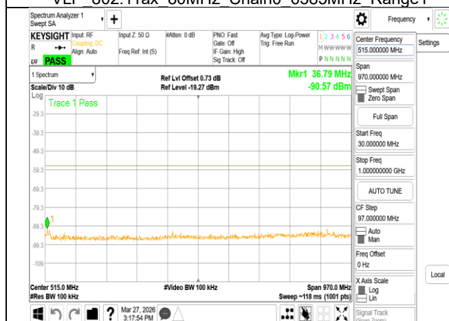
VLP 802.11ax 80MHz Chain1 5985MHz Range1
