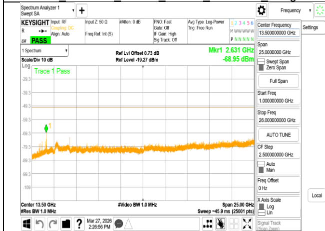
VLP 802.11ac 40MHz Chain1 6165MHz Range2
