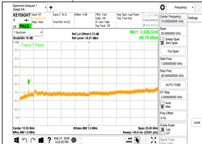
VLP 802.11ax 80MHz Chain1 6145MHz Range2
