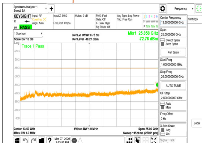
VLP 802.11be 20MHz Chain0 5955MHz Range2
