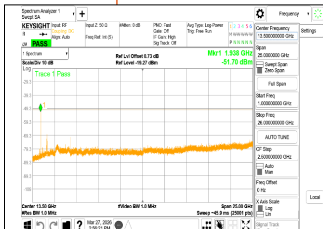
VLP_802.11ac_160MHz_Chain1_6185MHz_Range2
