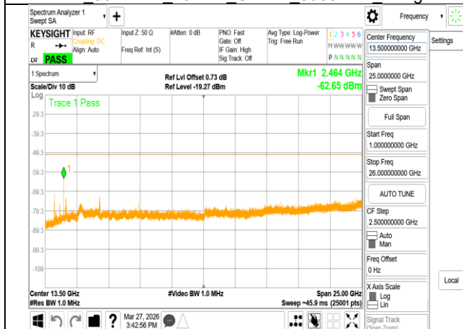
VLP 802.11be 40MHz Chain1 6165MHz Range2
