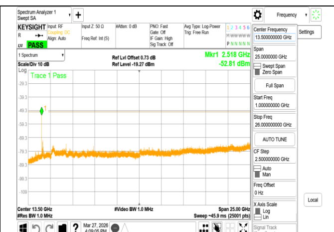
VLP 802.11be 320MHz Chain1 6265MHz Range2
