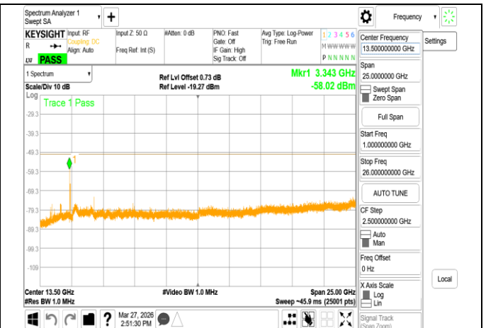
VLP_802.11ac_160MHz_Chain0_6025MHz_Range2
