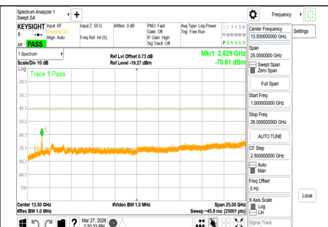
VLP 802.11ac 40MHz Chain1 6405MHz Range2
