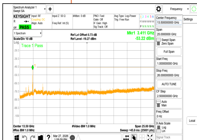
VLP 802.11n 40MHz Chain1 5965MHz Range2
