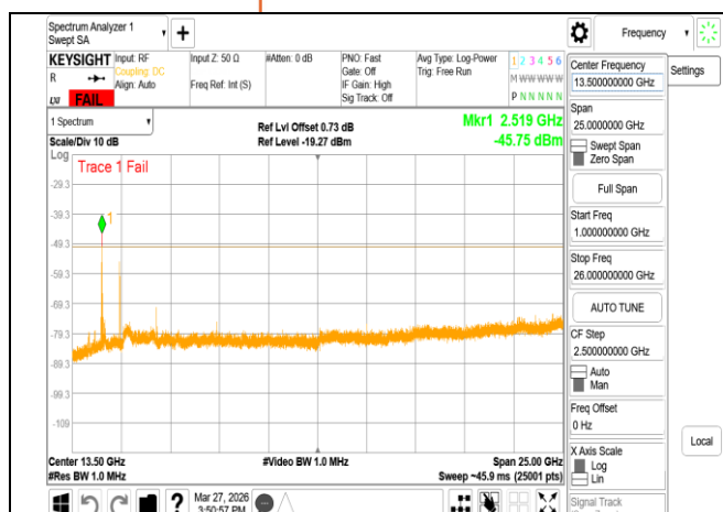
VLP 802.11be 80MHz Chain0 6145MHz Range2
