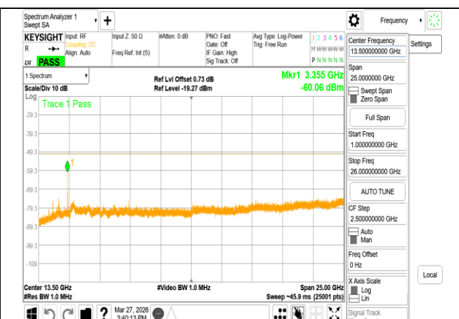
VLP 802.11be 40MHz Chain0 5965MHz Range2
