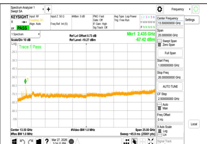
VLP 802.11ax 80MHz Chain0 6385MHz Range2
