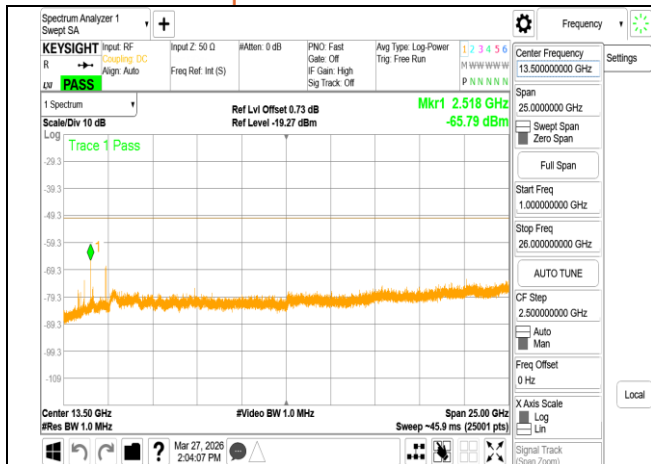
VLP 802.11n 40MHz Chain0 6165MHz Range2
