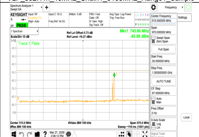
VLP 802.11n 40MHz Chain1 6405MHz Range1
