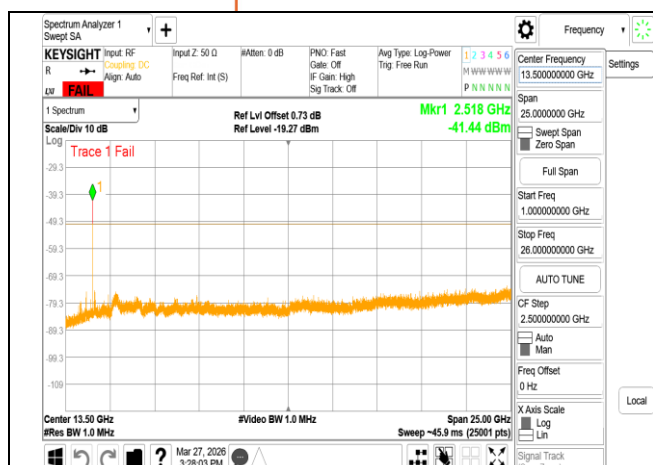
VLP_802.11ax_160MHz_Chain0_6185MHz_Range2
