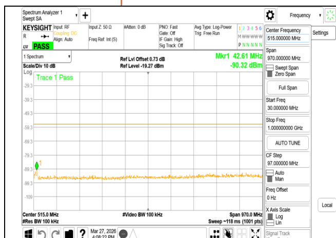
VLP 802.11be 320MHz Chain1 6265MHz Range1
