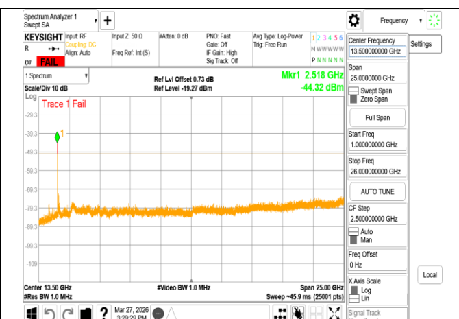
VLP_802.11ax_160MHz_Chain1_6185MHz_Range2
