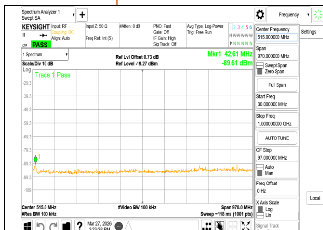
VLP 802.11ax 80MHz Chain0 6385MHz Range1
