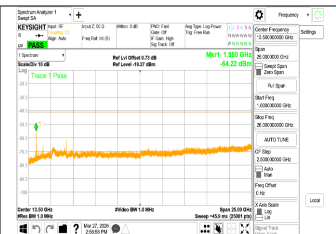
VLP_802.11ac_160MHz_Chain0_6345MHz_Range2
