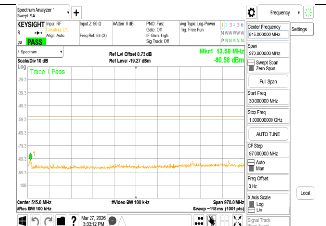
VLP_802.11be_20MHz_Chain0_5955MHz_Range1
