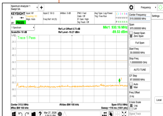
VLP 802.11be 40MHz Chain0 5965MHz Range1
