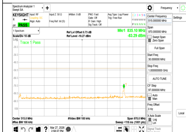
VLP_802.11ac_160MHz_Chain1_6345MHz_Range1
