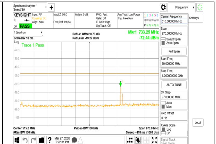
VLP 802.11ac 40MHz Chain1 5965MHz Range1
