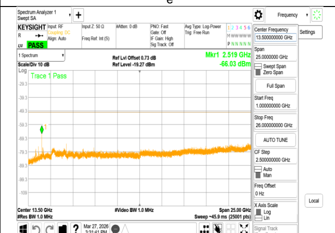
VLP_802.11ax_160MHz_Chain0_6345MHz_Range2
