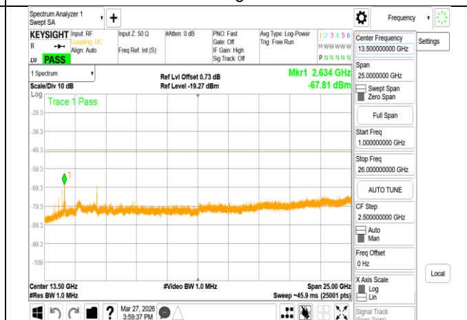
VLP_802.11be_160MHz_Chain1_6025MHz_Range2
