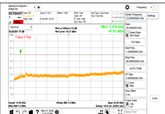
VLP 802.11ax 80MHz Chain0 5985MHz Range2
