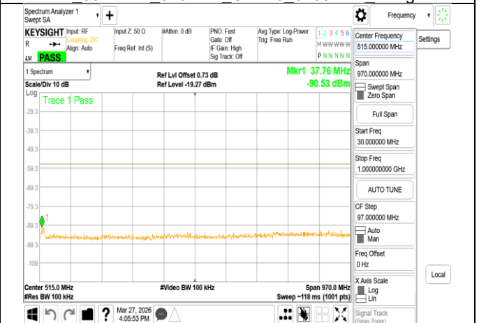
VLP_802.11be_320MHz_Chain1_6105MHz_Range1
