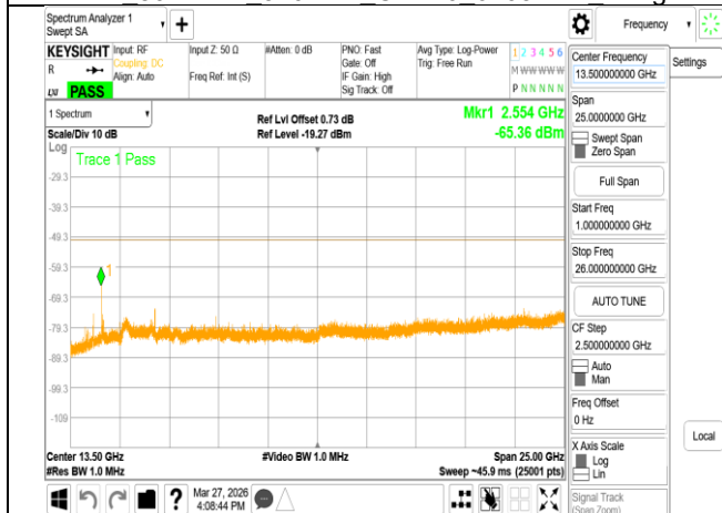
VLP_802.11be_320MHz_Chain0_6265MHz_Range2
