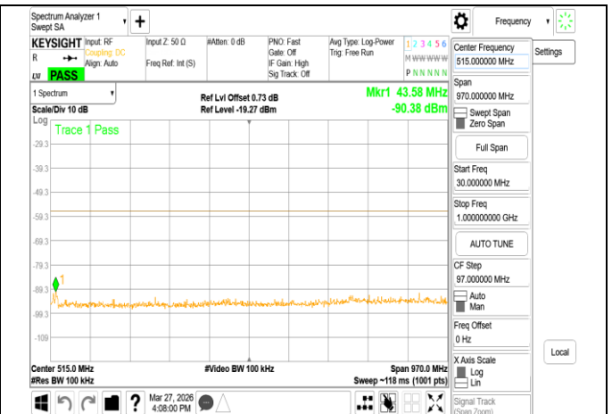
VLP_802.11be_320MHz_Chain0_6265MHz_Range1
