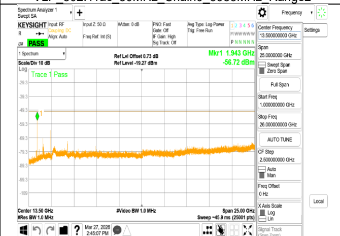
VLP 802.11ac 80MHz Chain0 6145MHz Range2
