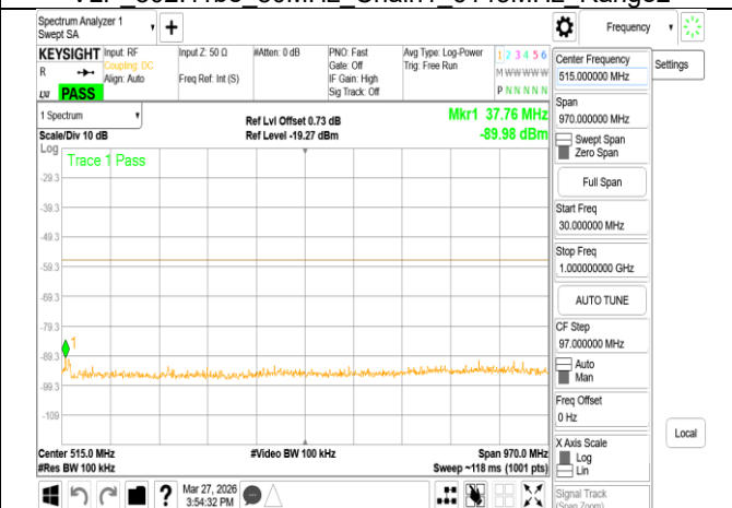
VLP 802.11be 80MHz Chain1 6385MHz Range1
