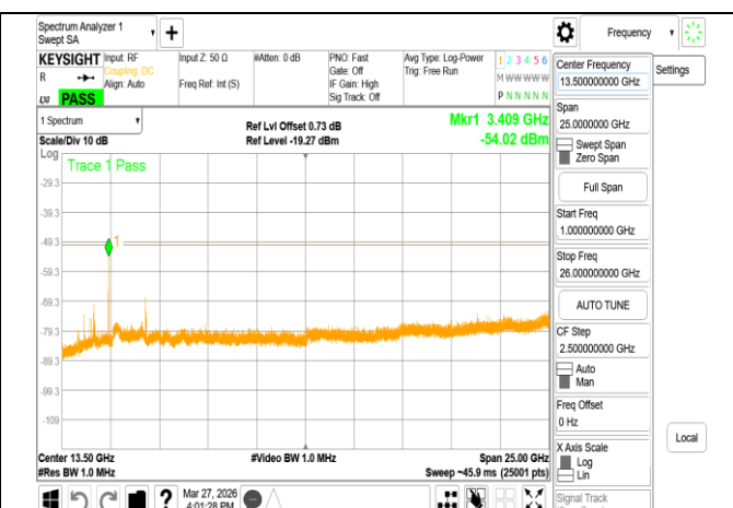
VLP_802.11be_160MHz_Chain1_6185MHz_Range2
