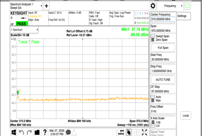
VLP_802.11ac_160MHz_Chain0_6185MHz_Range1
