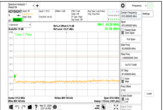
VLP 802.11ax 20MHz Chain1 6415MHz Range1
