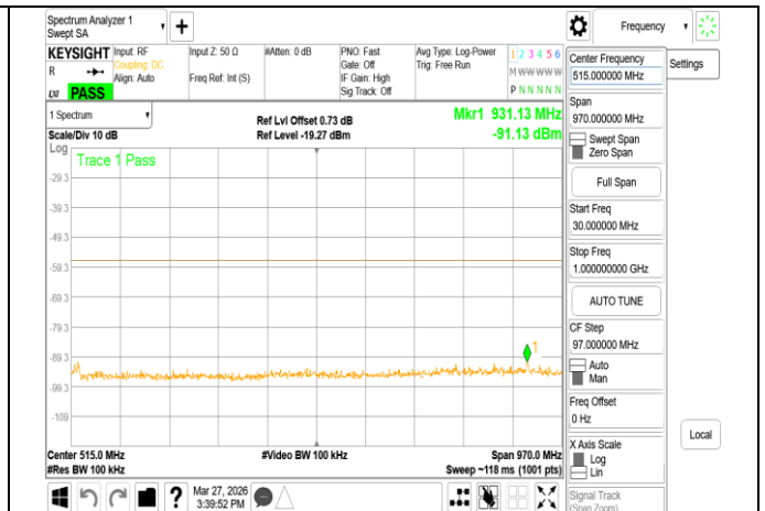
VLP 802.11be 40MHz Chain1 5965MHz Range1
