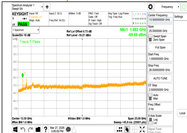
VLP 802.11ax 20MHz Chain1 6175MHz Range2
