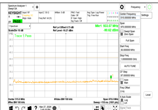
VLP 802.11ac 80MHz Chain0 6385MHz Range1
