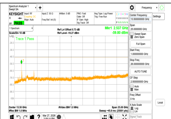
VLP 802.11n 40MHz Chain1 6405MHz Range2
