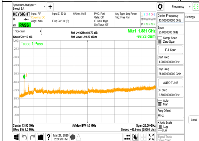
VLP 802.11ac 40MHz Chain1 5965MHz Range2
