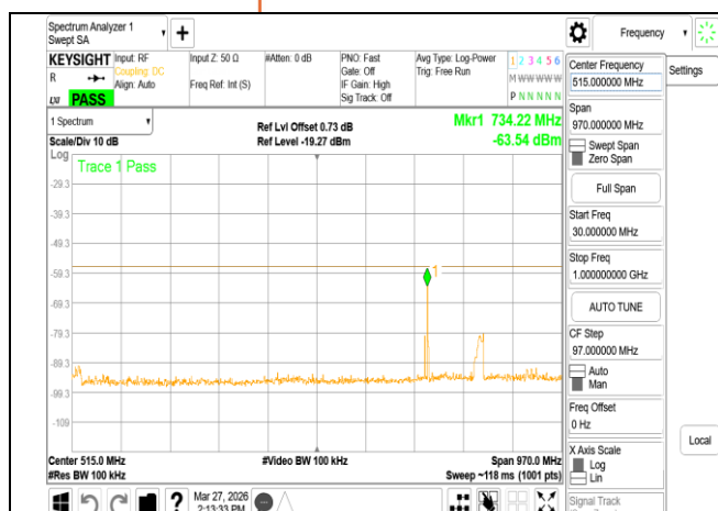
VLP_802.11ac_20MHz_Chain0_6175MHz_Range1
