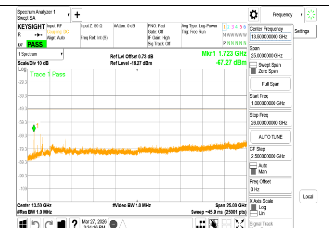
VLP 802.11be 20MHz Chain1 5955MHz Range2
