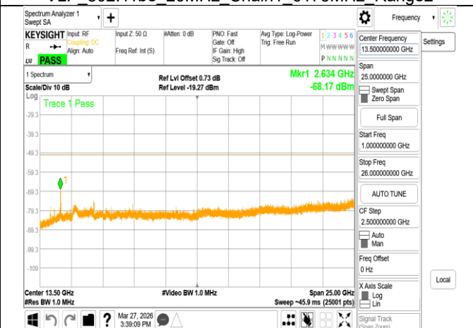
VLP 802.11be 20MHz Chain1 6415MHz Range2
