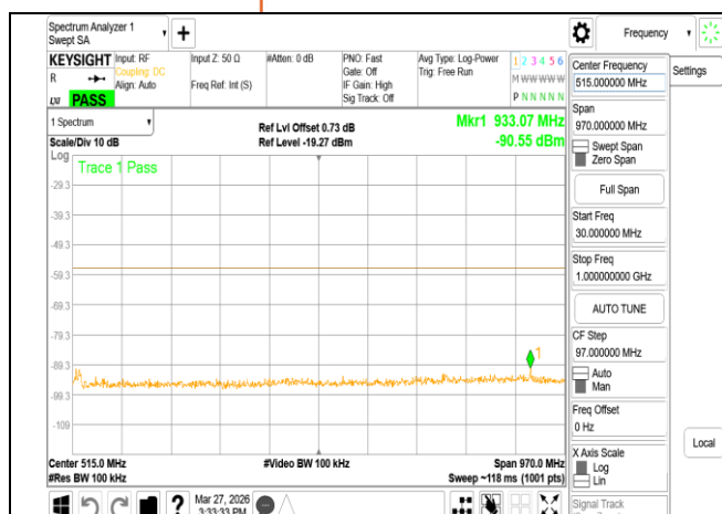
VLP 802.11be 20MHz Chain1 5955MHz Range1
