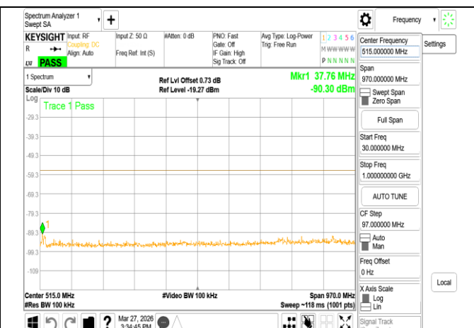
VLP 802.11be 20MHz Chain0 6175MHz Range1
