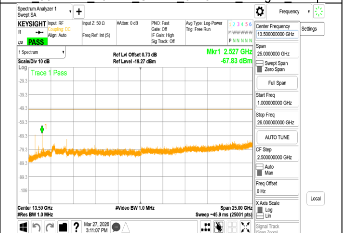
VLP 802.11ax 40MHz Chain0 5965MHz Range2
