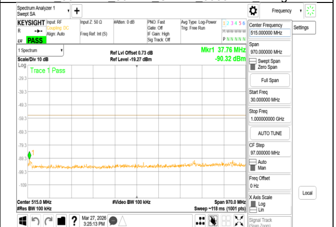
VLP 802.11ax 160MHz Chain0 6025MHz Range1
