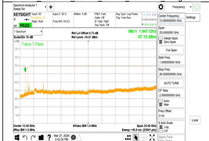
VLP 802.11ac 80MHz Chain1 5985MHz Range2
