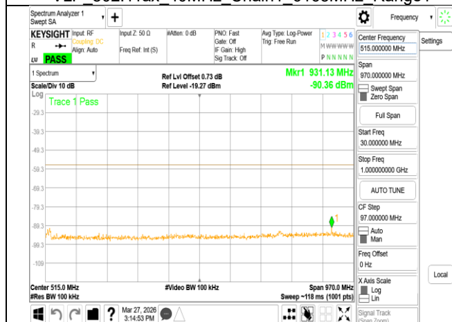
VLP 802.11ax 40MHz Chain1 6405MHz Range1
