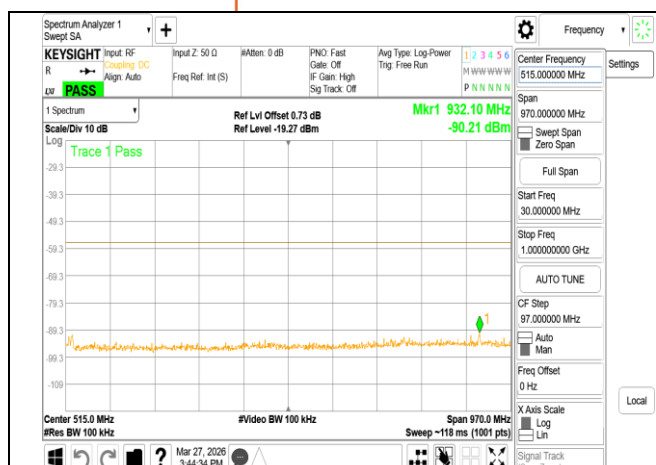
VLP 802.11be 40MHz Chain1 6405MHz Range1
