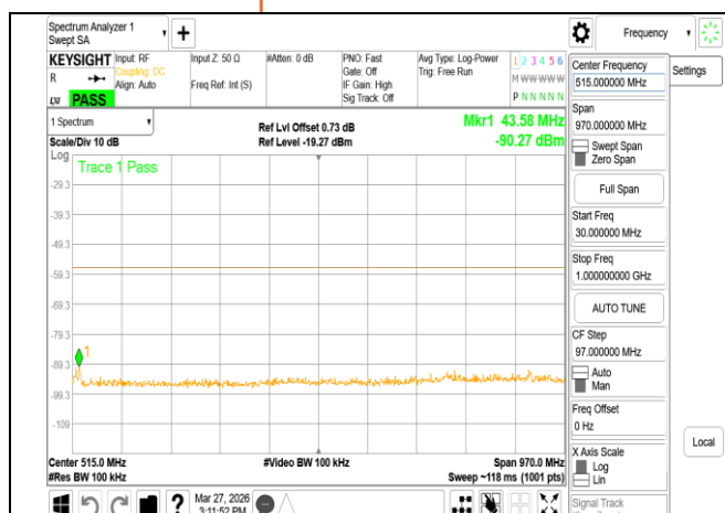
VLP 802.11ax 40MHz Chain0 6165MHz Range1
