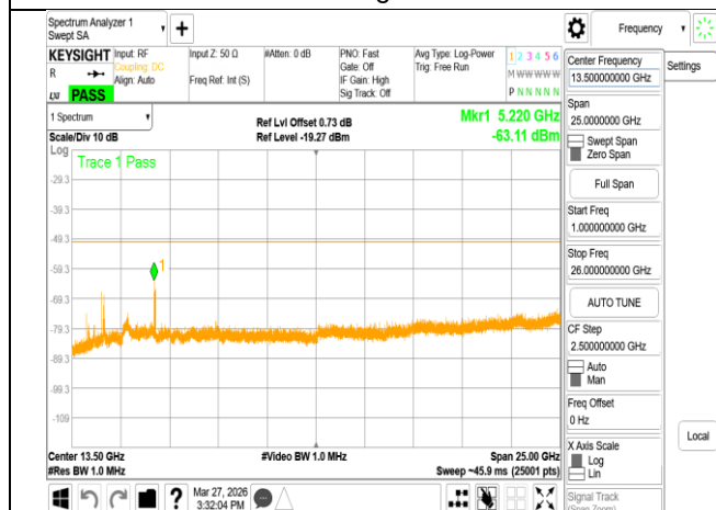
VLP_802.11ax_160MHz_Chain1_6345MHz_Range2
