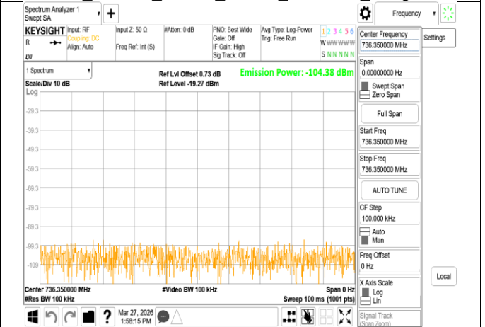
VLP 802.11n 40MHz Chain1 5965MHz Range1 Sample
