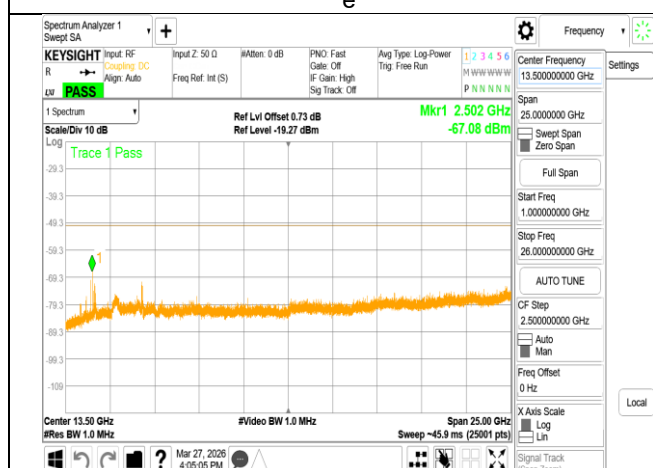
VLP_802.11be_160MHz_Chain1_6345MHz_Range2
