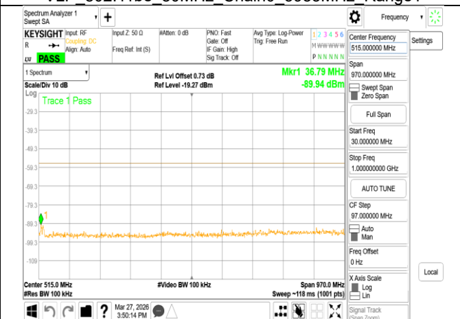
VLP 802.11be 80MHz Chain0 6145MHz Range1
