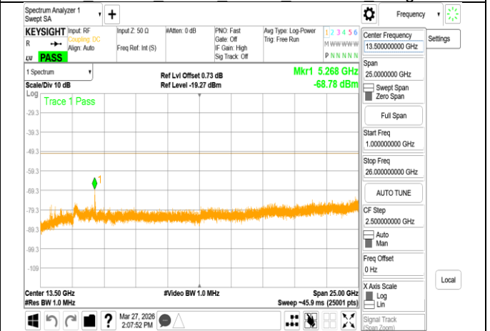
VLP 802.11n 40MHz Chain0 6405MHz Range2
