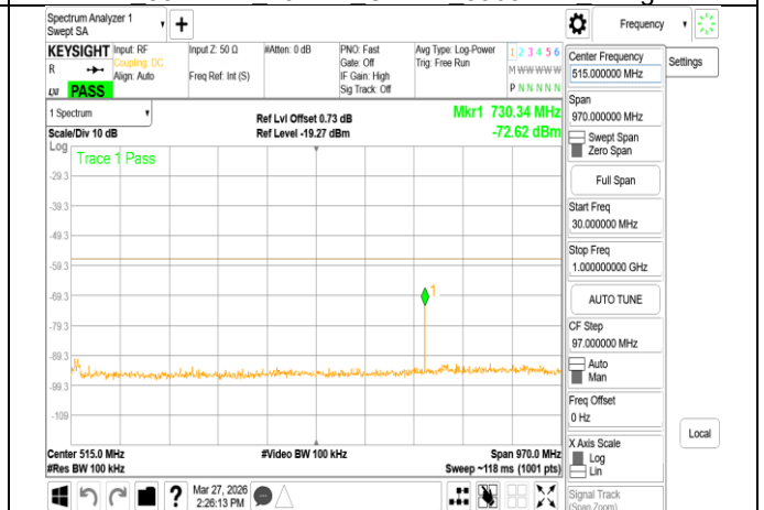
VLP 802.11ac 40MHz Chain1 6165MHz Range1
