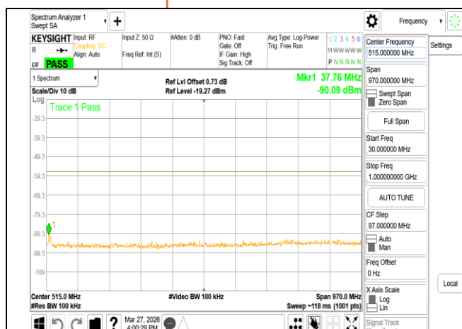
VLP_802.11be_160MHz_Chain1_6185MHz_Range1
