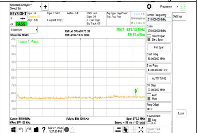
VLP 802.11ax 160MHz Chain0 6185MHz Range1
