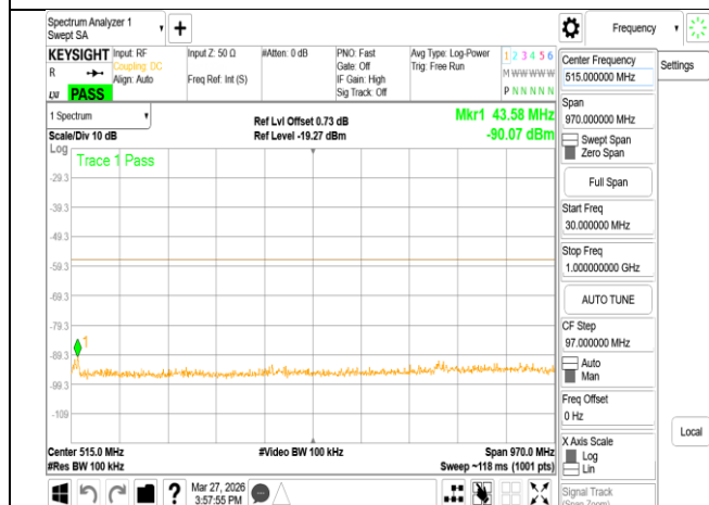
VLP_802.11be_160MHz_Chain1_6025MHz_Range1
