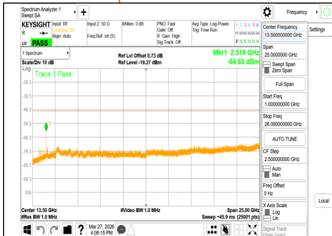
VLP_802.11be_320MHz_Chain0_6105MHz_Range2
