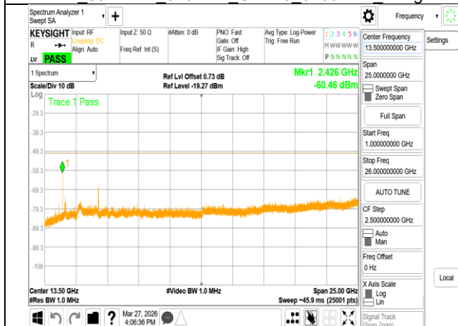
VLP_802.11be_320MHz_Chain1_6105MHz_Range2
