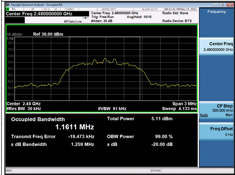
Test_Graph_EDR_ANT1_2480_3Mbps_OBW
