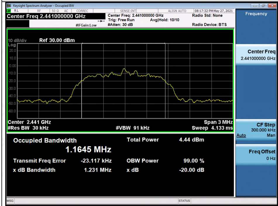
Test_Graph_EDR_ANT1_2441_2Mbps_OBW
