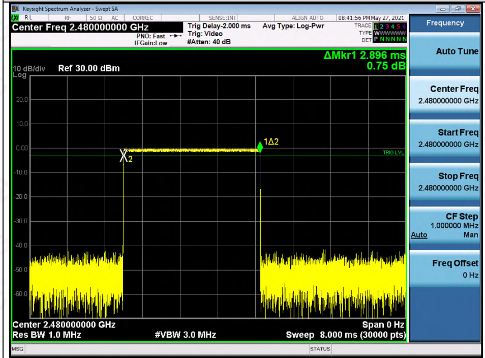
Test_Graph_BR_HOP_ANT1_NA_1Mbps_2480_Time per Burst
