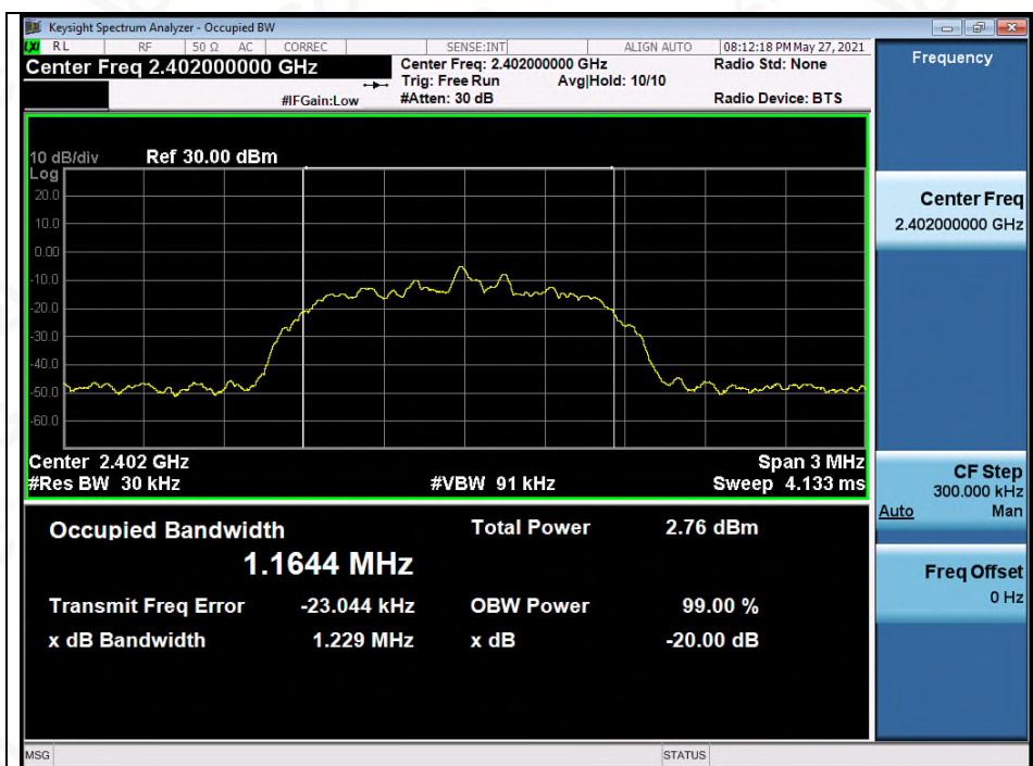
Test_Graph_EDR_ANT1_2402_2Mbps_OBW
