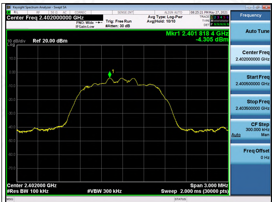
Test_Graph_EDR_ANT1_2402_3Mbps_Reference Level
