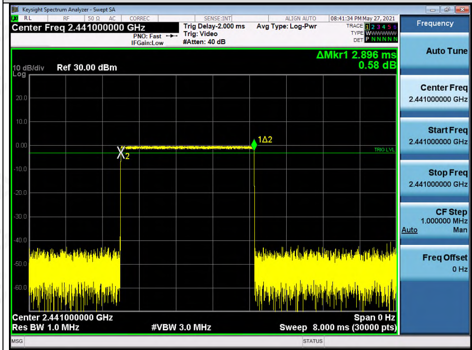
Test_Graph_BR_HOP_ANT1_NA_1Mbps_2441_Time per Burst
