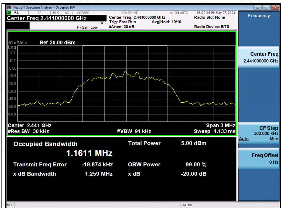
Test_Graph_EDR_ANT1_2441_3Mbps_OBW
