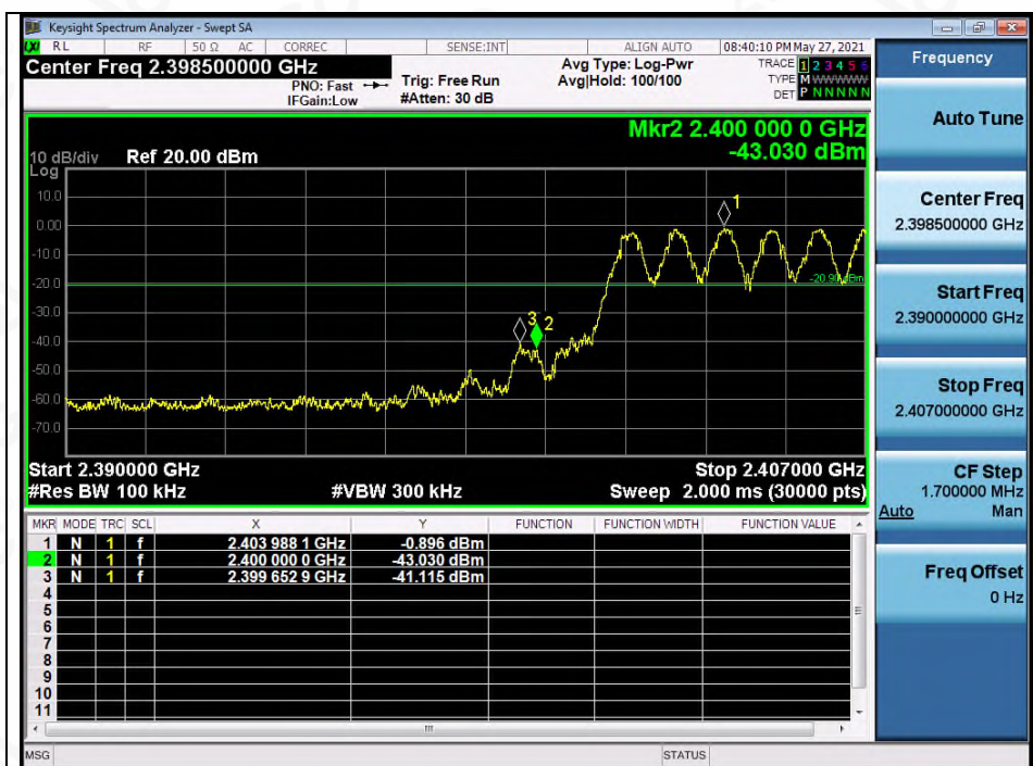
Test_Graph_BR_HOP_ANT1_NA_1Mbps_Lower Band Edge Emissions
