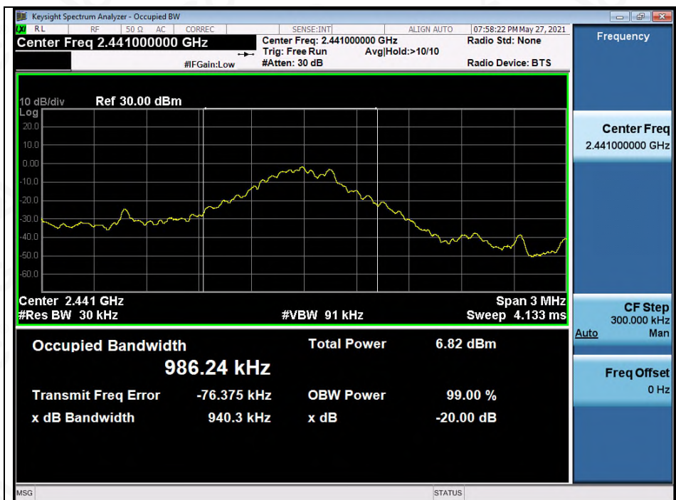
Test_Graph_BR_ANT1_2441_1Mbps_OBW
