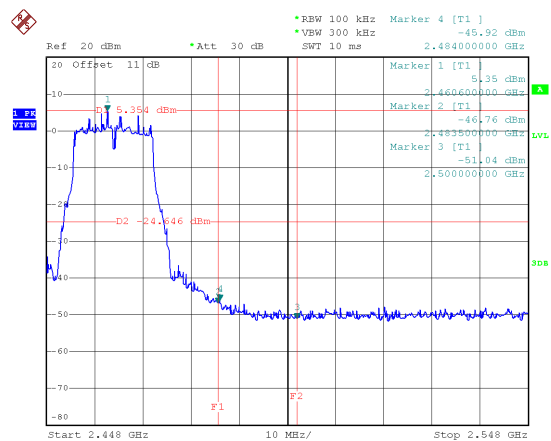
IEEE 802.11g 頻帶範圍外(上邊緣頻帶)之任意 100 kHz 內最大射頻功率
