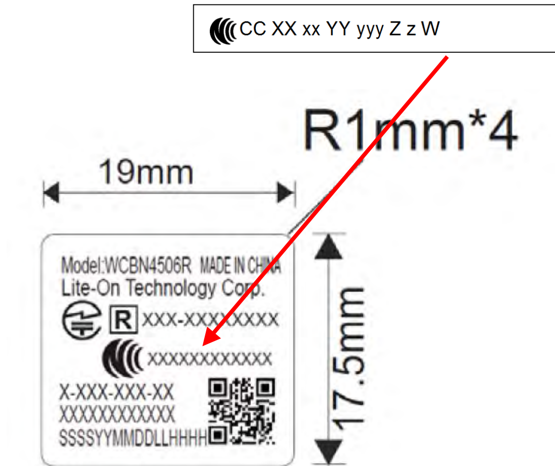
Label 位置圖
