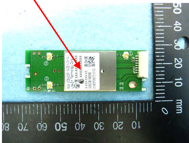
Label 位置圖
