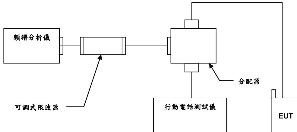
測試架構圖(傳導量測方式):
