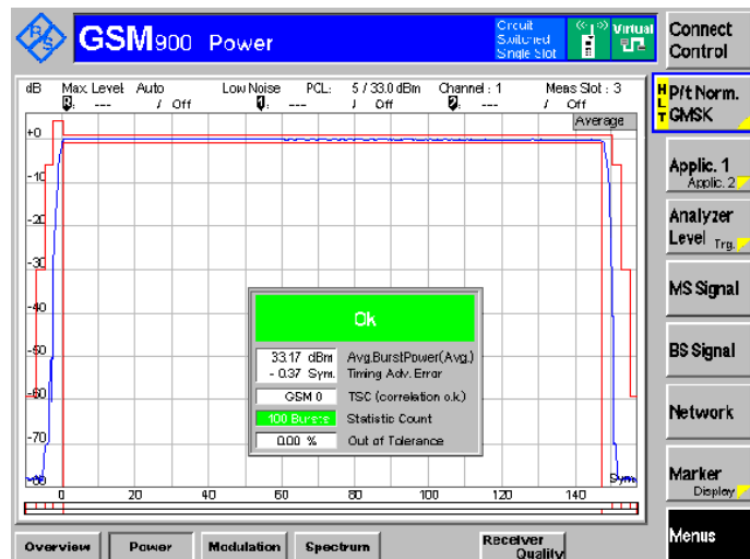
GSM900常壓-常溫叢訊功率/時間關係圖
