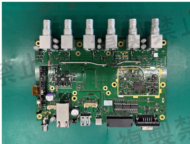
RF 基板_表面_電源基板有,シールドケース有
