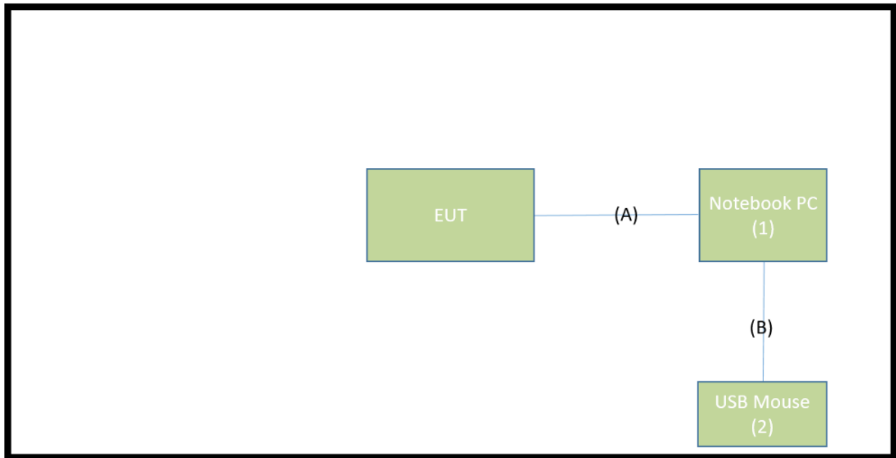
待測物測試配置圖 Mode1~Mode4
