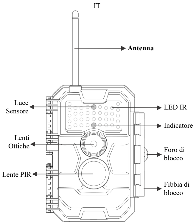
Figura 1: Vista frontale
