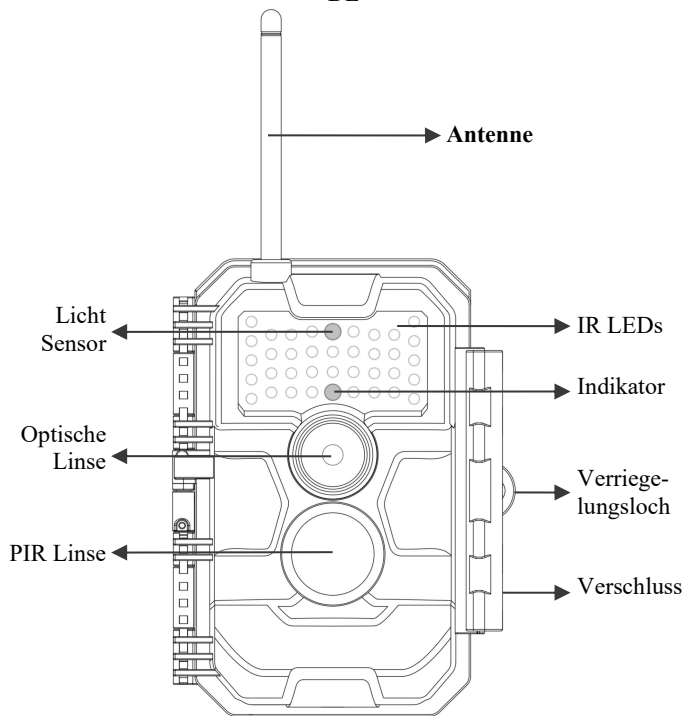
Abb. 1: Vorderansicht
