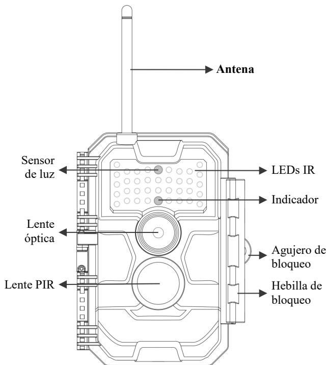
Figura 1: Vista frontal
