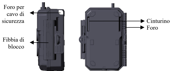
Figura 3: Vista destra/posteriore
