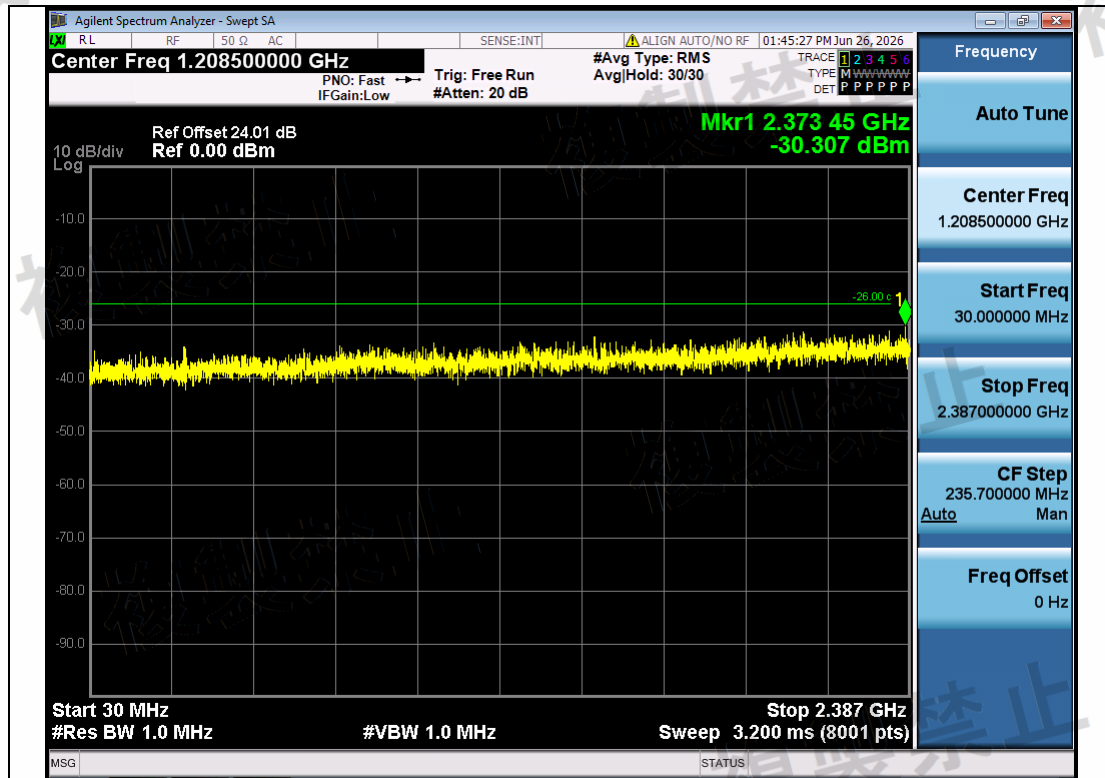
NTNV-11B-Ant1-2412-30~2387-PASS
