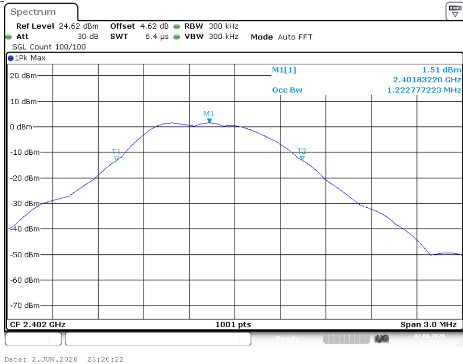
OBW NVNT BLE 1M 2402MHz Ant1
