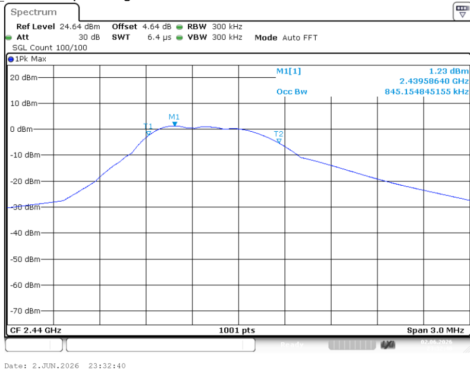
Spreading Bandwidth NVNT BLE 1M 2440MHz Ant1
