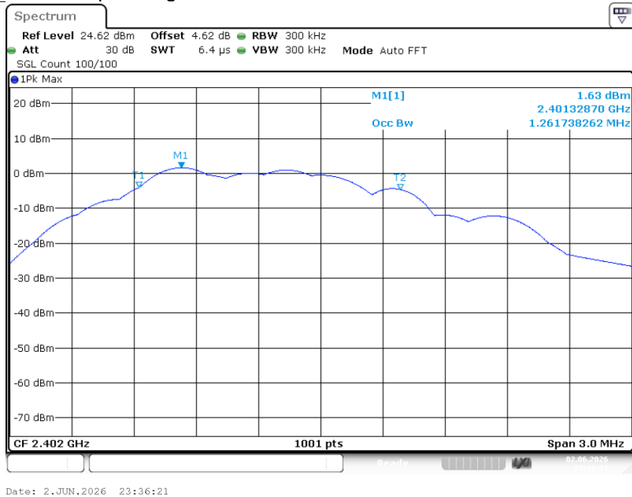
Spreading Bandwidth NVNT BLE 2M 2402MHz Ant1
