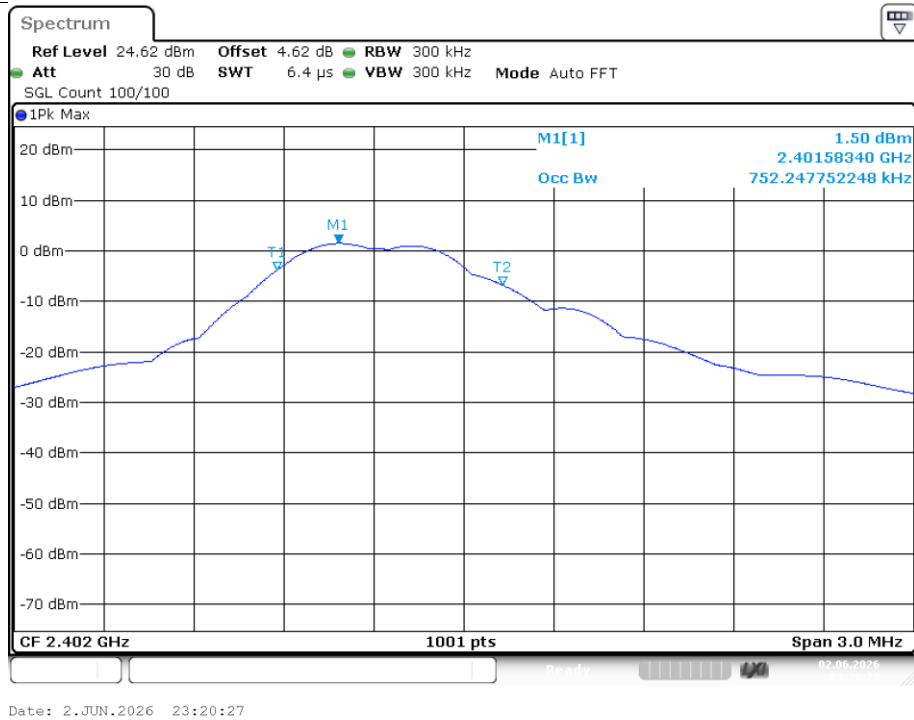
Spreading Bandwidth NVNT BLE 1M 2402MHz Ant1
