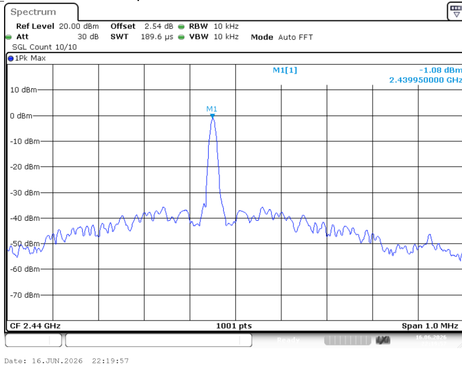
Freq. Error NVNT BLE 2440MHz Ant1
