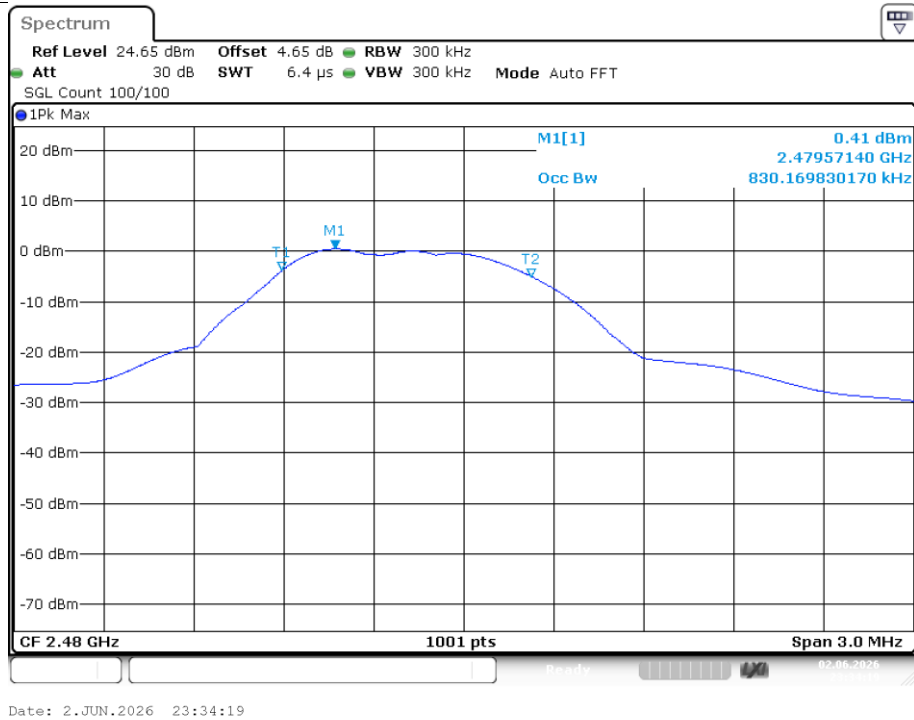
Spreading Bandwidth NVNT BLE 1M 2480MHz Ant1
