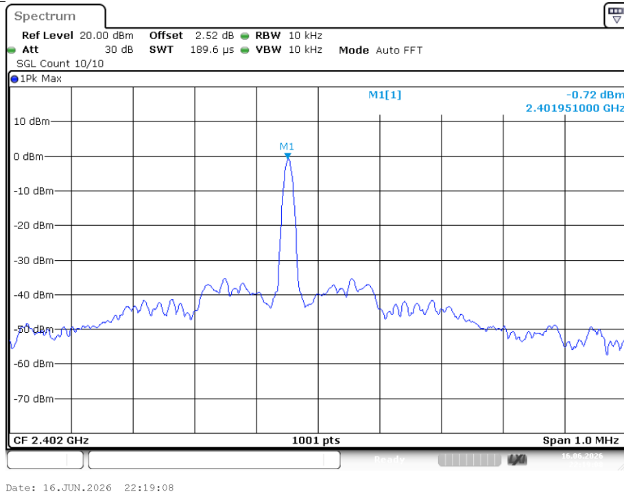
Freq. Error NVNT BLE 2402MHz Ant1
