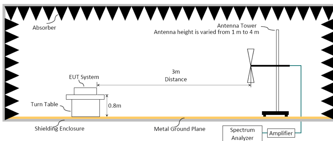
圖 2: 量測頻率高於 1GHz 之測試配置
