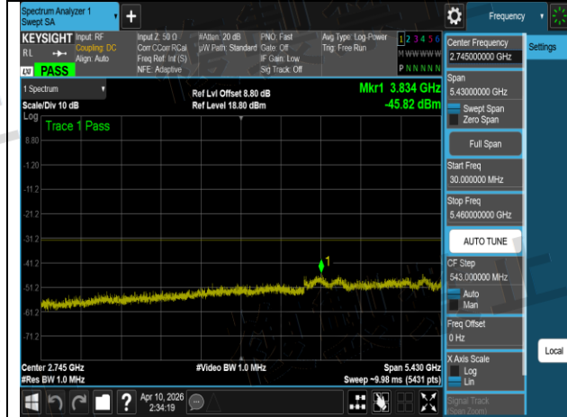
W56 802.11a 20MHz Chain3 5600MHz 1
