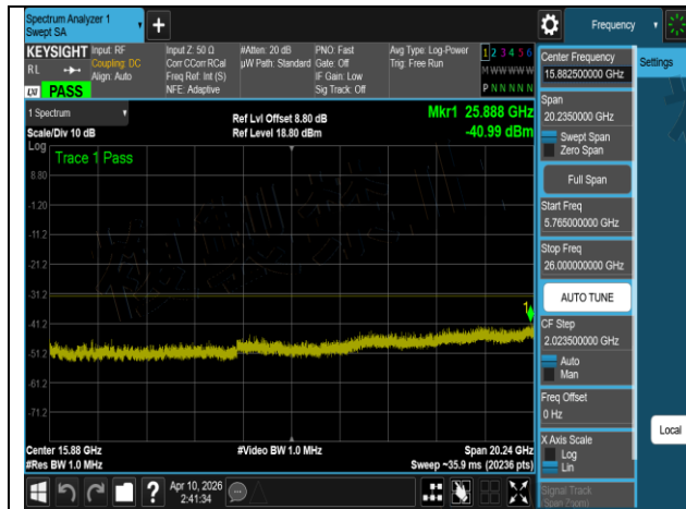
W56 802.11a 20MHz Chain3 5600MHz 4
