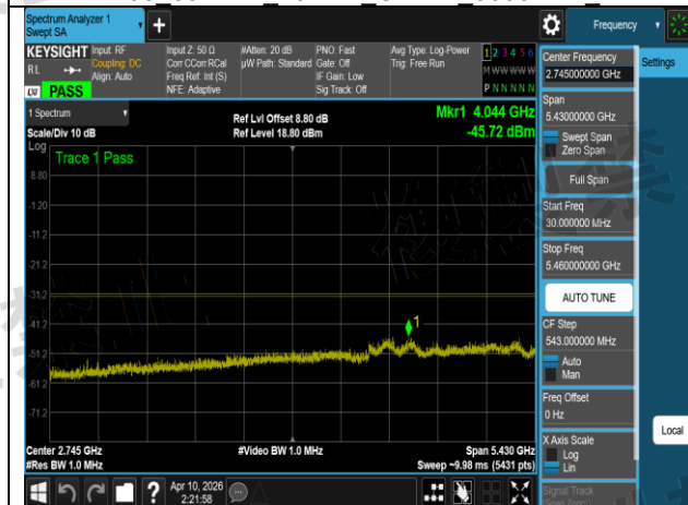
W56 802.11a 20MHz Chain2 5500MHz 1
