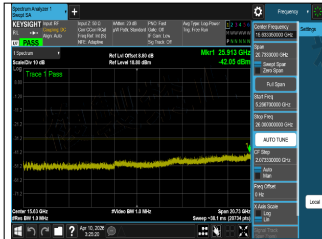
W52 802.11ax 20MHz Chain2 5220MHz 7
