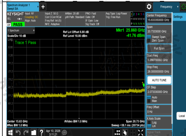
W52 802.11ax 20MHz Chain3 5180MHz 7
