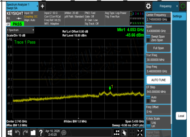
W56 802.11a 20MHz Chain1 5720MHz 1
