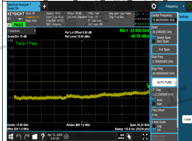
W56 802.11a 20MHz Chain3 5720MHz 4
