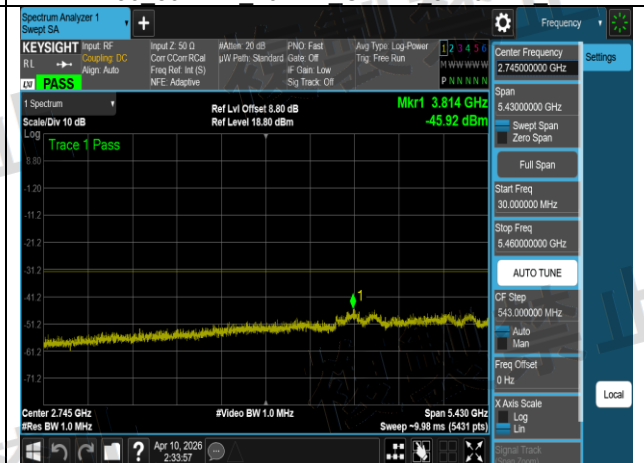
W56 802.11a 20MHz Chain2 5600MHz 1
