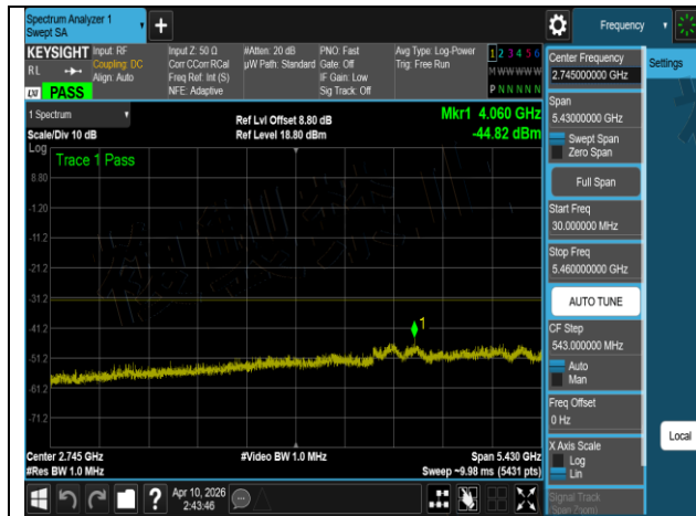
W56 802.11a 20MHz Chain2 5720MHz 1
