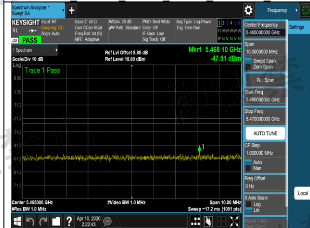
W56 802.11a 20MHz Chain0 5500MHz 2
