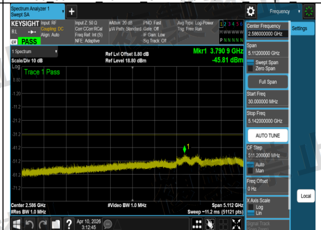
W52 802.11ax 20MHz Chain0 5220MHz 1
