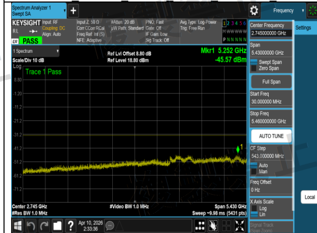
W56 802.11a 20MHz Chain1 5600MHz 1
