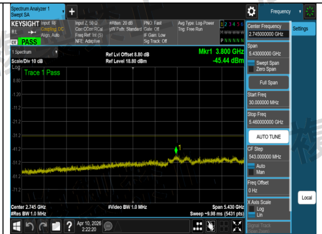
W56 802.11a 20MHz Chain3 5500MHz 1
