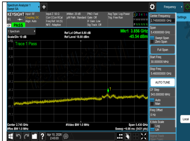
W56 802.11a 20MHz Chain0 5720MHz 1
