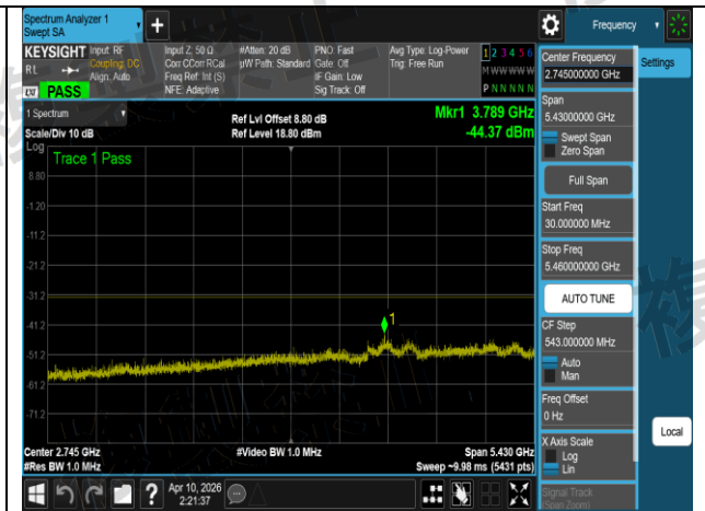
W56 802.11a 20MHz Chain1 5500MHz 1
