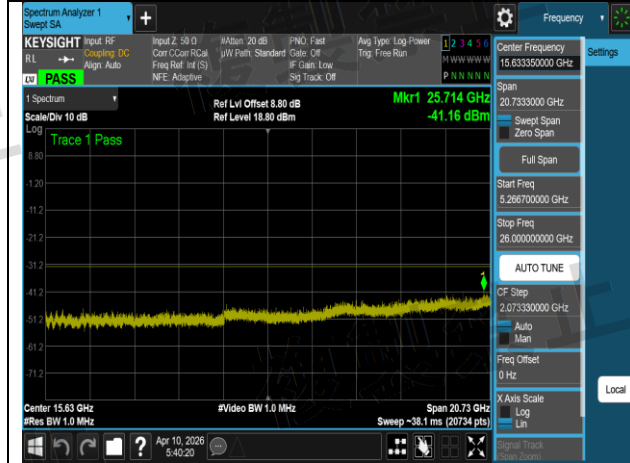
W52 802.11ax 20MHz Chain2 5240MHz 7
