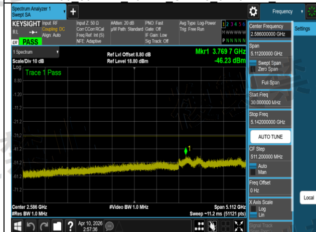
W52 802.11ax 20MHz Chain0 5180MHz 1
