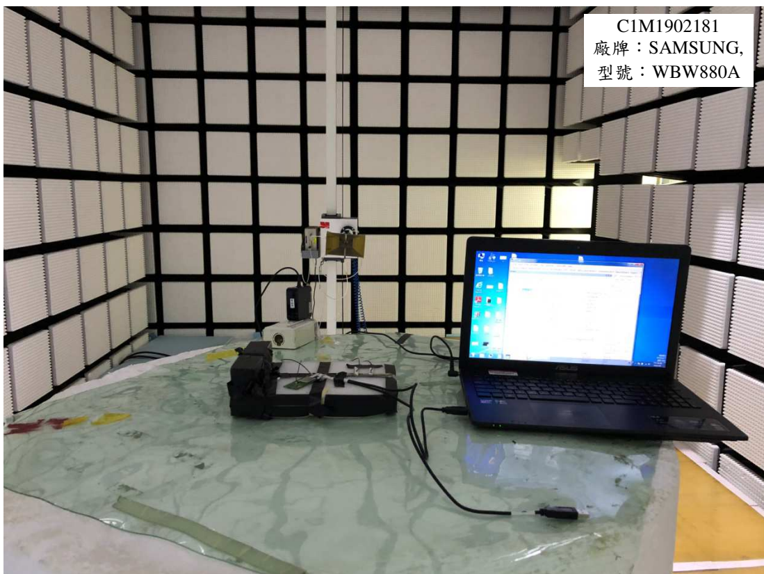
2.2. 量測頻率高於 1GHz 之測試 平放
