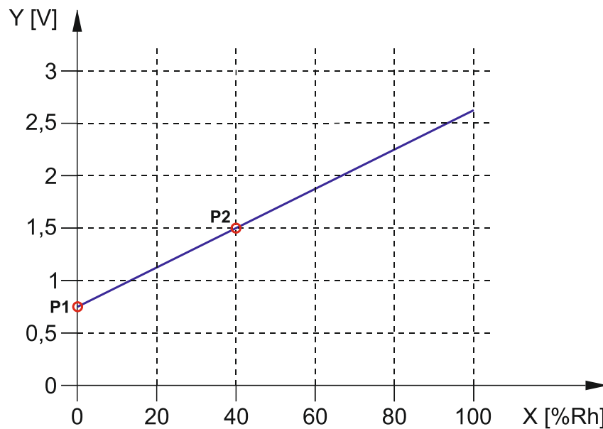
Abb. 22. Beispiel für lineare Kennlinie des Luftfeuchtesensors. X – relative Feuchte [% Rh], Y – Spannung am Ausgang des Sensors [V].
