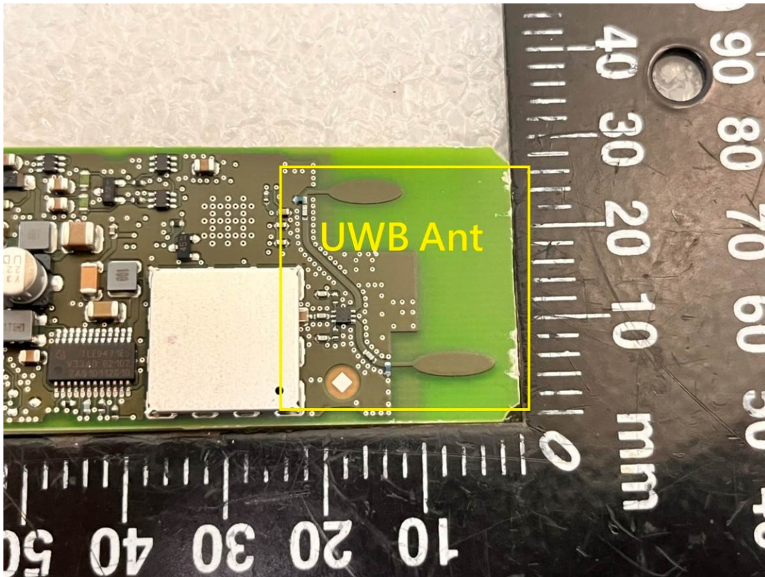
EUT-20. UWB Ant
