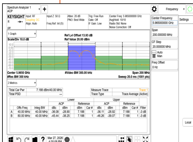
VLP 802.11ac 40MHz 5965MHz Combine
