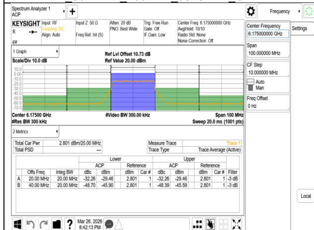
VLP 802.11be 20MHz Chain0 6175MHz
