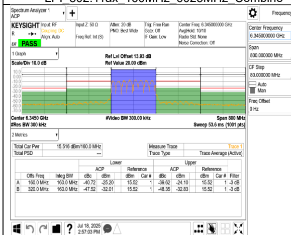
LPI 802.11ax 160MHz 6345MHz Combine
