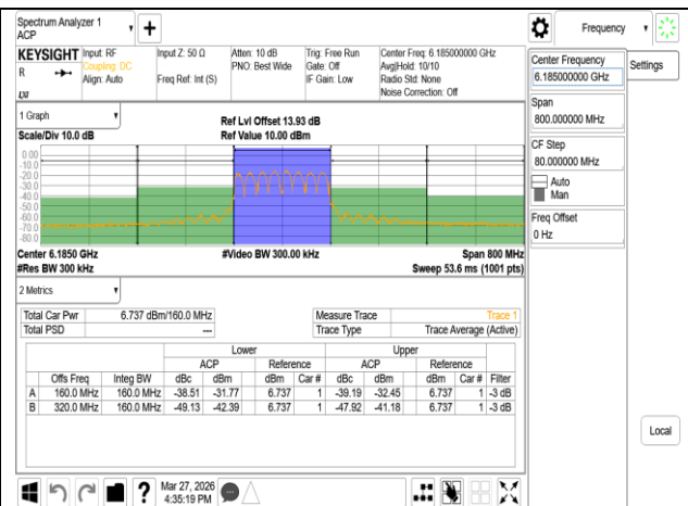
VLP 802.11ac 160MHz 6185MHz Combine
