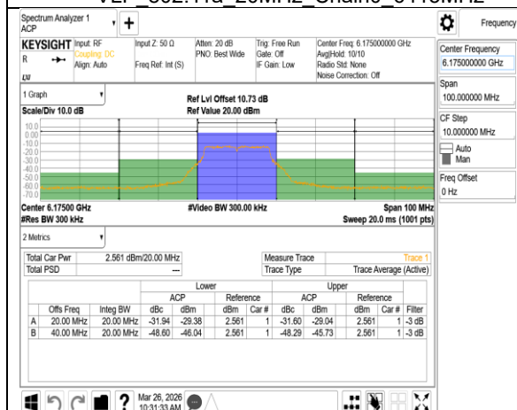
VLP 802.11a 20MHz Chain1 6175MHz
