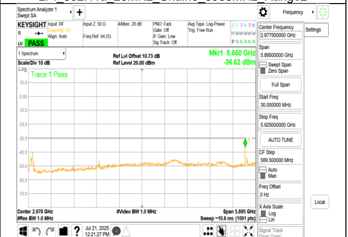
LPI 802.11a 20MHz Chain0 6175MHz Range1
