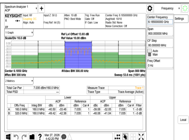
VLP 802.11ax 160MHz 6185MHz Combine
