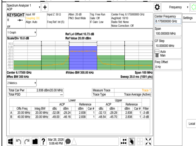
VLP 802.11ax 20MHz Chain0 6175MHz
