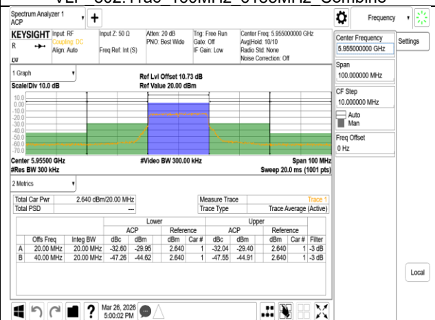
VLP 802.11ax 20MHz Chain0 5955MHz
