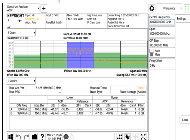
VLP 802.11ax 160MHz 6025MHz Combine
