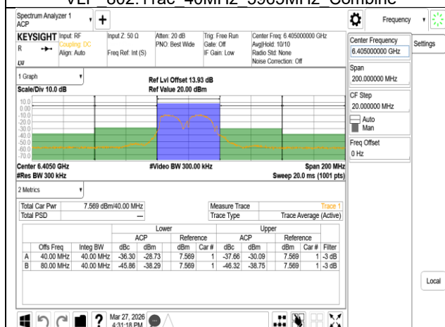
VLP 802.11ac 40MHz 6405MHz Combine
