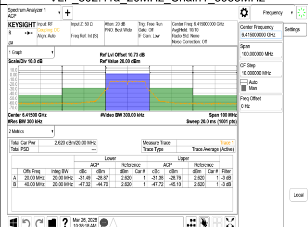
VLP 802.11a 20MHz Chain1 6415MHz
