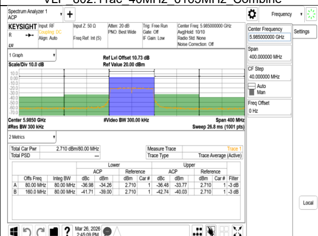
VLP 802.11ac 80MHz Chain0 5985MHz
