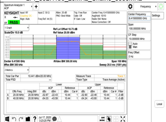
LPI 802.11be 20MHz Chain0 6415MHz
