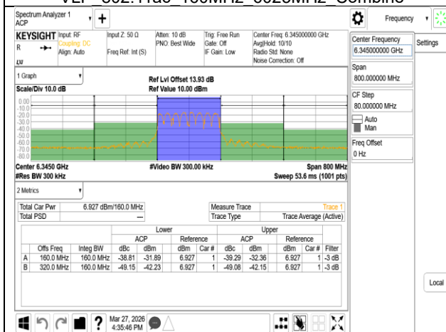
VLP 802.11ac 160MHz 6345MHz Combine
