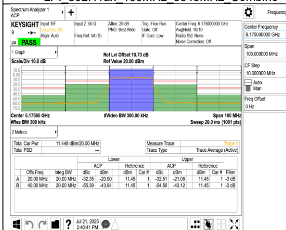
LPI 802.11be 20MHz Chain0 6175MHz
