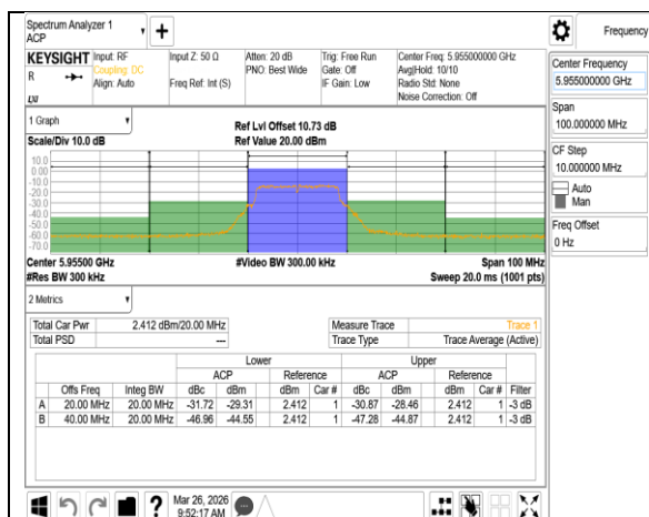
VLP 802.11a 20MHz Chain0 5955MHz
