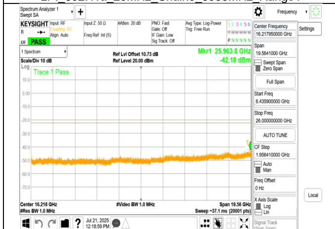
LPI 802.11a 20MHz Chain0 5955MHz Range3
