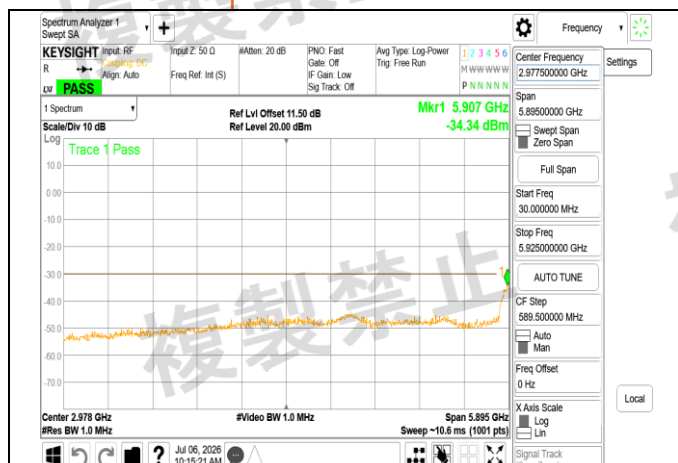
LPI 802.11ax 160MHz Chain0 6025MHz Range1
