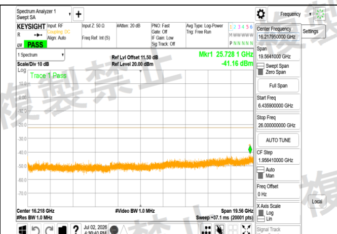
LPI 802.11ax 20MHz Chain1 6415MHz Range3
