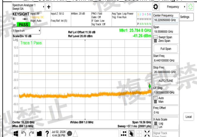
LPI 802.11ax 40MHz Chain0 5965MHz Range3
