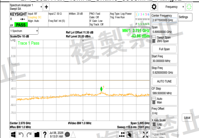
LPI 802.11ax 40MHz Chain0 6165MHz Range1
