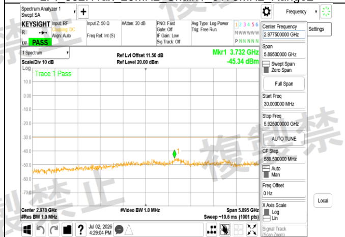
LPI 802.11ax 20MHz Chain1 6415MHz Range1
