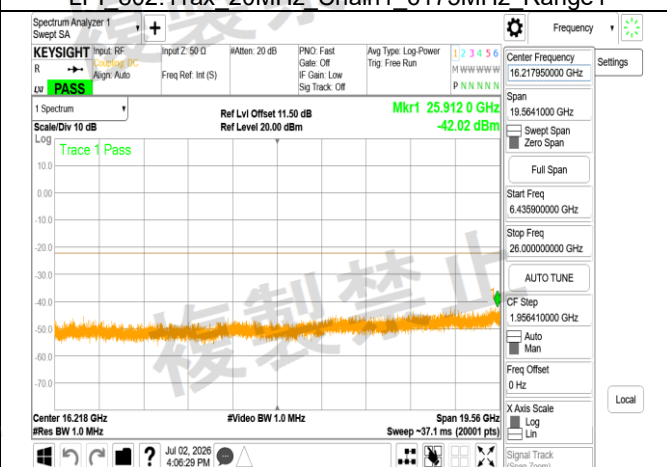
LPI 802.11ax 20MHz Chain1 6175MHz Range3
