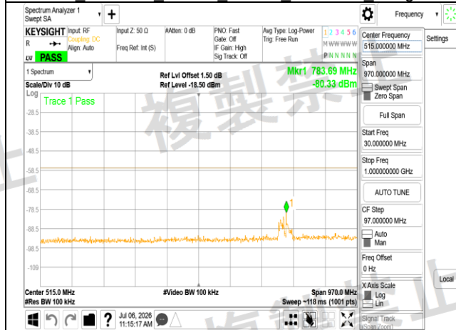
LPI 802.11ac 80MHz Chain0 6145MHz Range1
