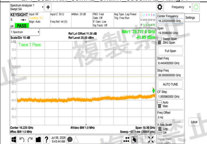
LPI 802.11ax 80MHz Chain1 5985MHz Range3
