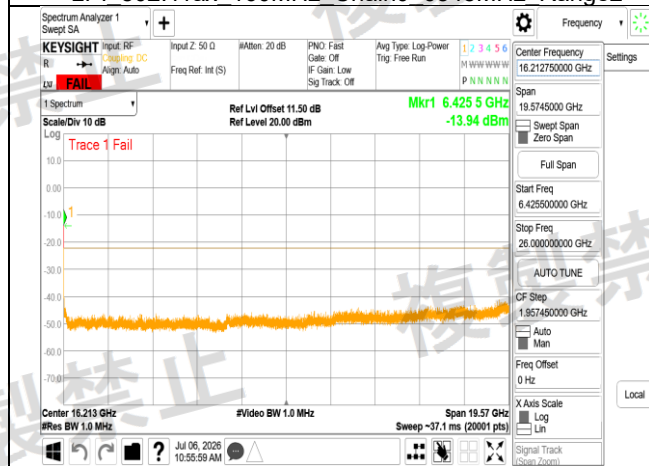
LPI 802.11ax 160MHz Chain0_6345MHz Range3
