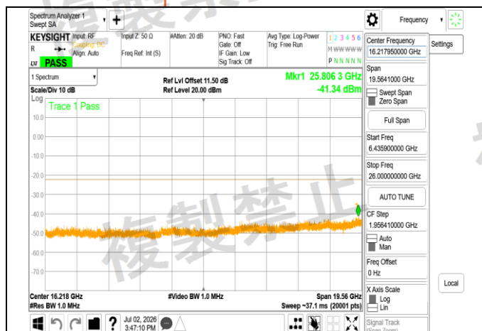
LPI 802.11ax 20MHz Chain1 5955MHz Range3
