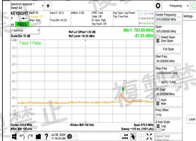
LPI 802.11ac 80MHz Chain0 6385MHz Range1
