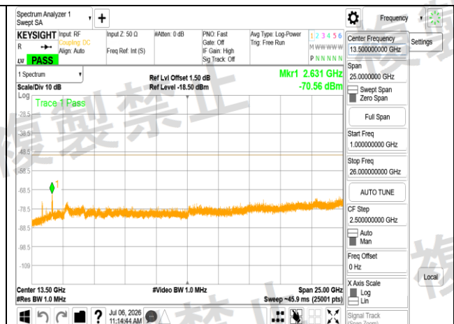
LPI 802.11ac 80MHz Chain0 5985MHz Range2
