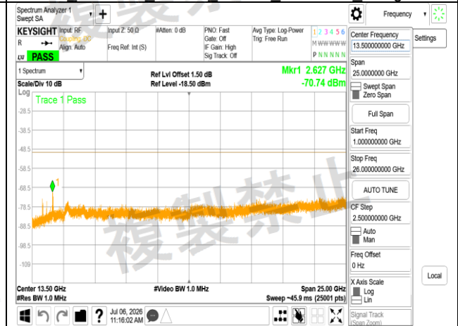
LPI 802.11ac 80MHz Chain0 6145MHz Range2
