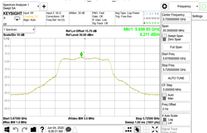
802.11a_20MHz_5700MHz
