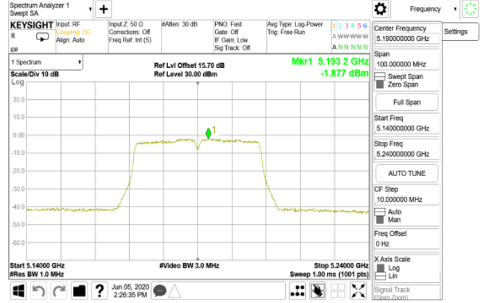
802.11n_40MHz_5190MHz
