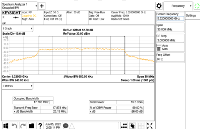
802.11n_20MHz_Chain1_5320MHz
