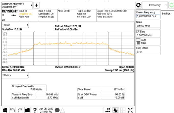
802.11n_20MHz_Chain1_5785MHz
