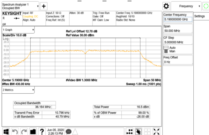
802.11n_40MHz_Chain1_5190MHz
