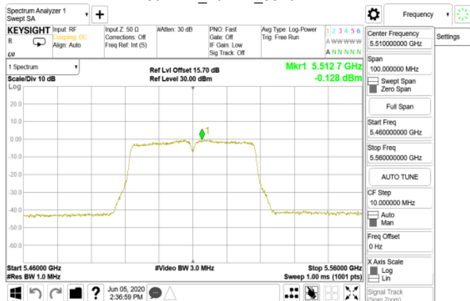
802.11n_40MHz_5510MHz
