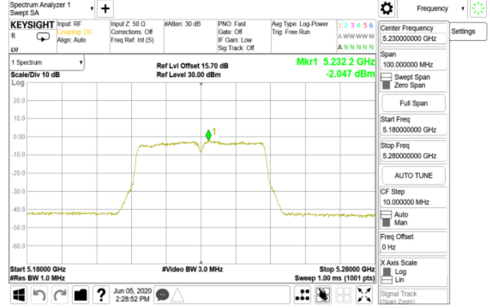
802.11n_40MHz_5230MHz
