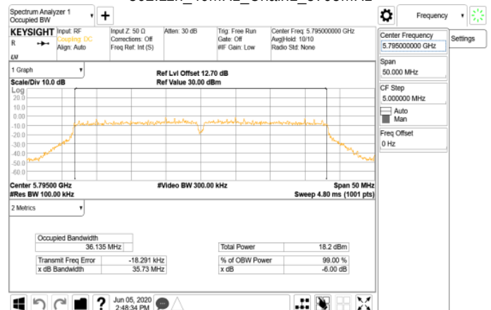
802.11n_40MHz_Chain1_5795MHz
