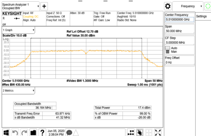
802.11n_40MHz_Chain0_5510MHz
