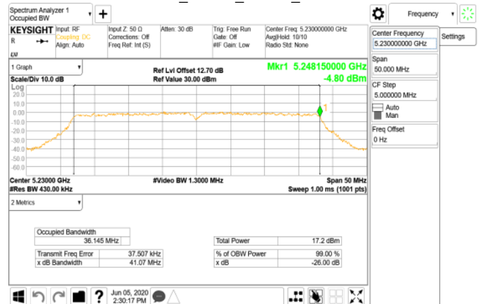
802.11n_40MHz_Chain0_5230MHz
