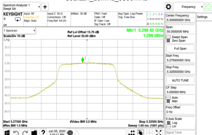
802.11n_20MHz_5300MHz
