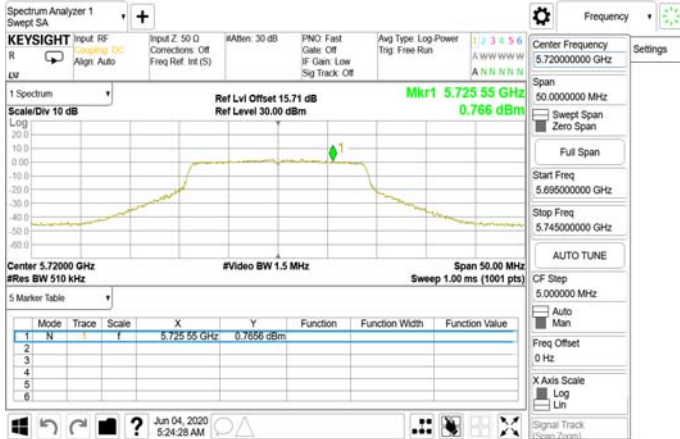
802.11n_20MHz_5720MHz
