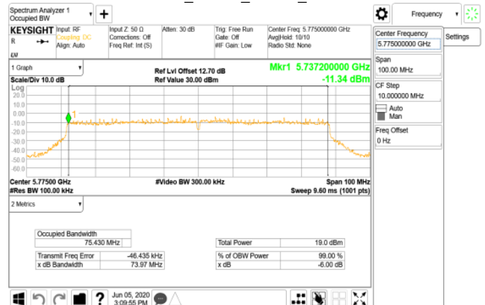
802.11ac_80MHz_Chain0_5775MHz
