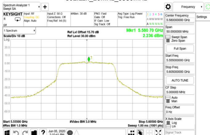
802.11n_20MHz_5580MHz
