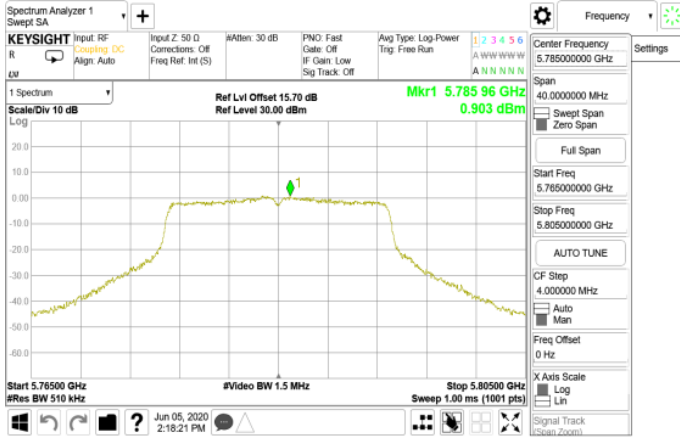
802.11n_20MHz_5785MHz
