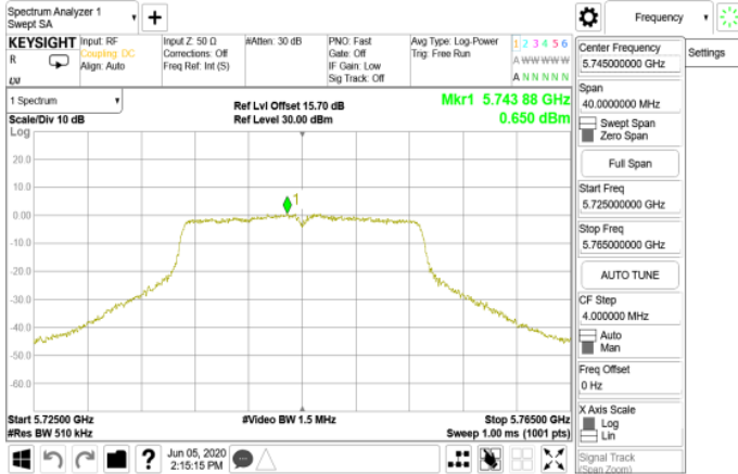
802.11n_20MHz_5745MHz
