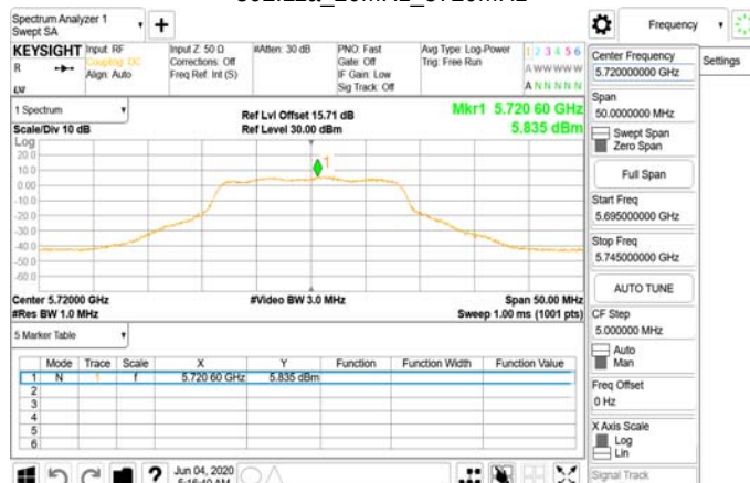
802.11a_20MHz_5720MHz
