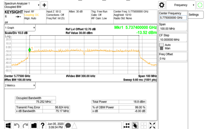
802.11ac_80MHz_Chain1_5775MHz
