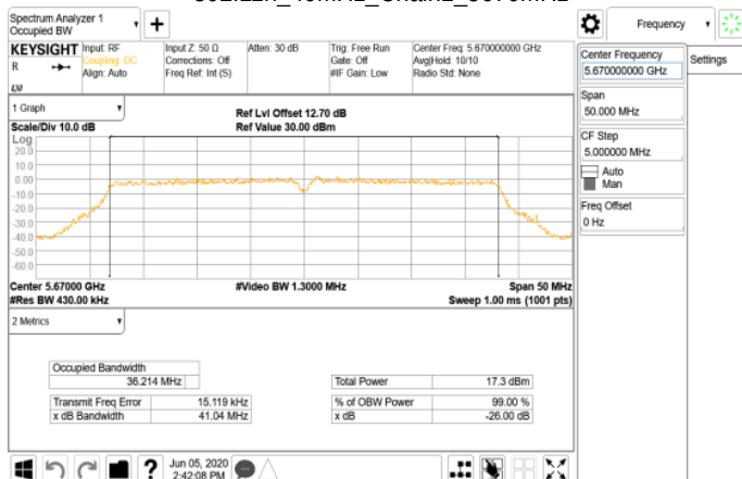
802.11n_40MHz_Chain1_5670MHz
