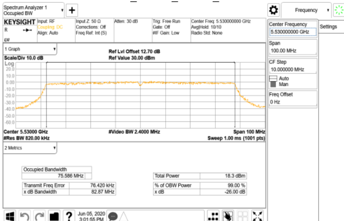
802.11ac_80MHz_Chain0_5530MHz
